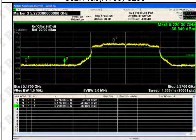
802.11ac(HT80)-5290
