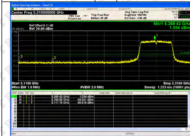
802.11ac(HT80)-5290
