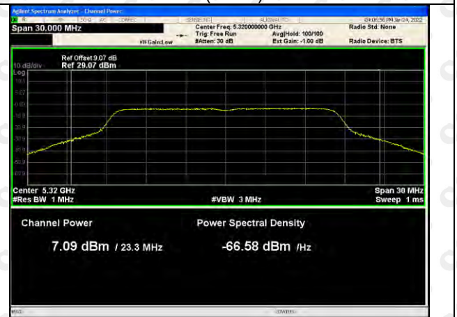
802.11ac(VH20)-5320
