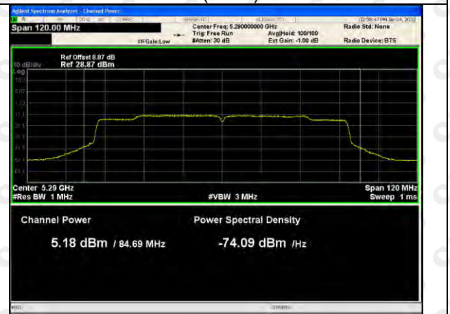
802.11ac(HT80)-5290
