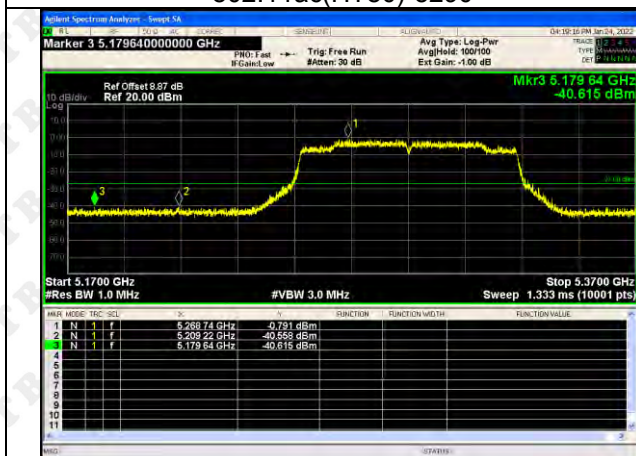
802.11ac(HT80)-5290
