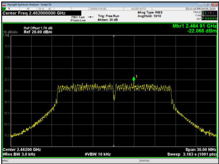
802.11g - CH11
