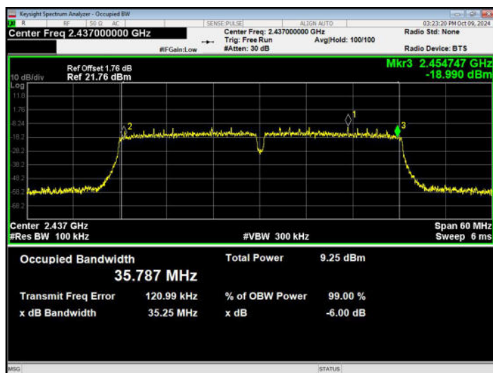
802.11n40 - CH06
