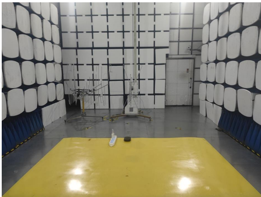
Fig. 1 (Below 1GHz)
