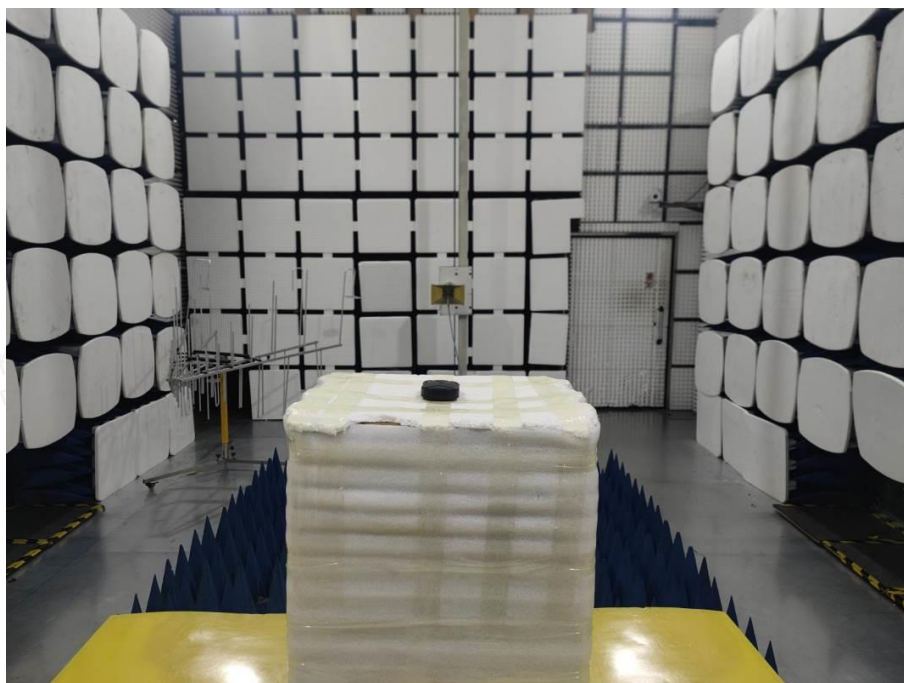
Fig. 2 (Above 1GHz)
