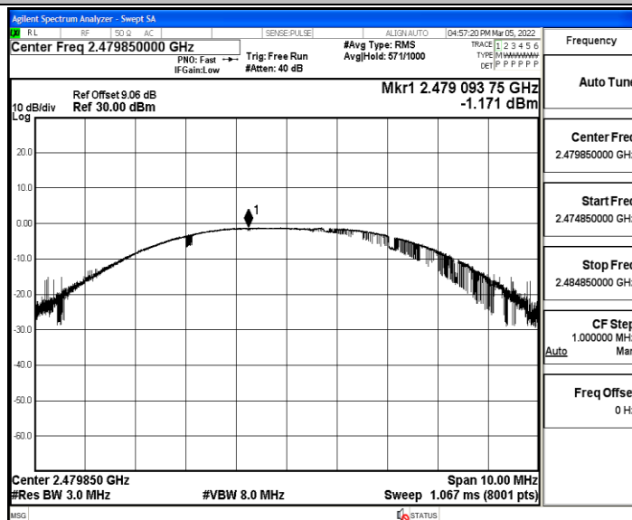
SRD_Ant1_2479.85
