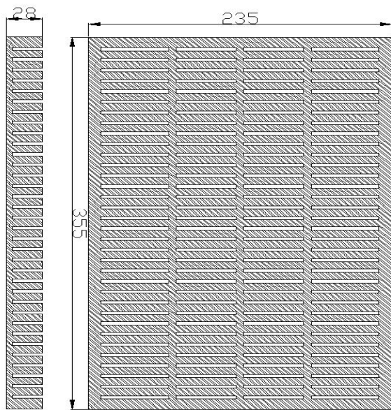
侧视图
