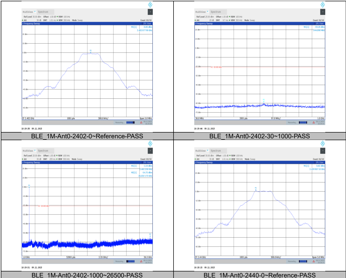
BLE 1M-Ant0-2402-1000~26500-PASS
