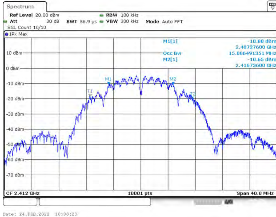
6dB NVNT 802.11b 2412MHz Ant1
