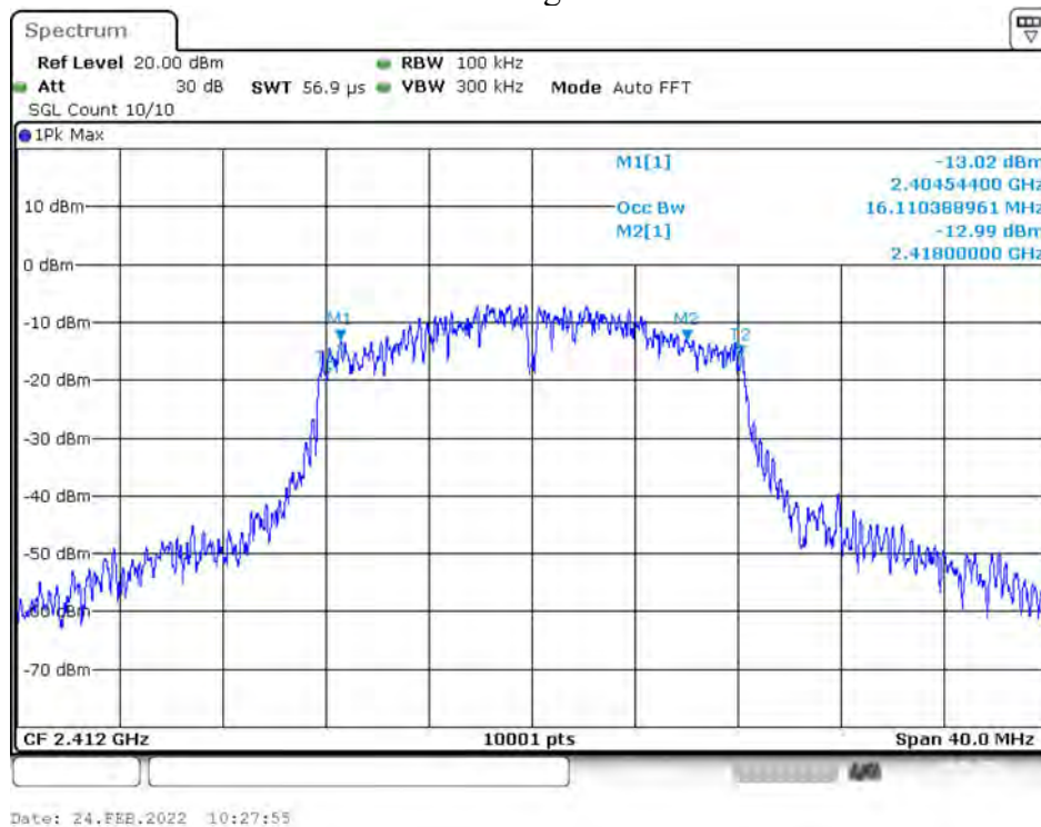
6dB NVNT 802.11g 2412MHz Ant1
