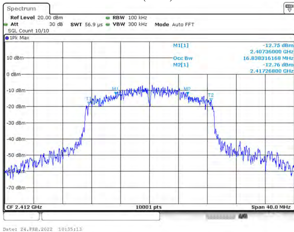
6dB NVNT 802.11n(HT20) 2412MHz Ant1
