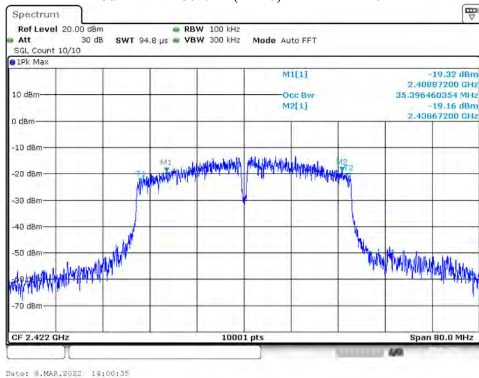
6dB NVNT 802.11n(HT40) 2422MHz Ant1
