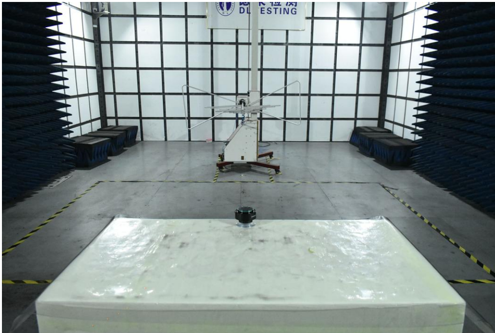
EUT TEST PHOTO
