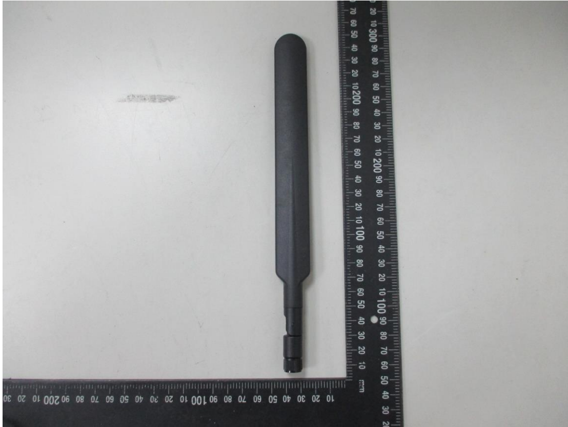
Antenna: SP-12K0915GS01-01
