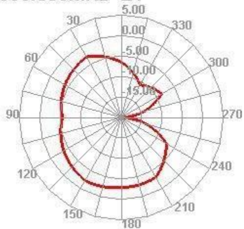
850.000MHz E1
