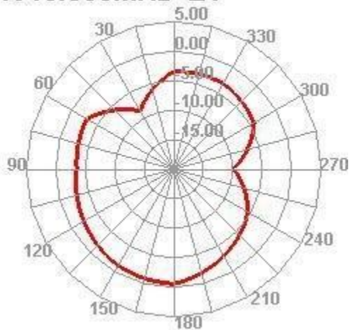
1910.000MHz E1
