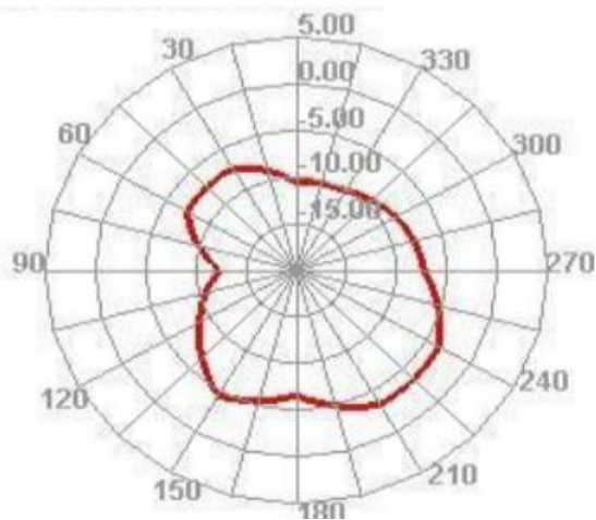
5250.000MHz
