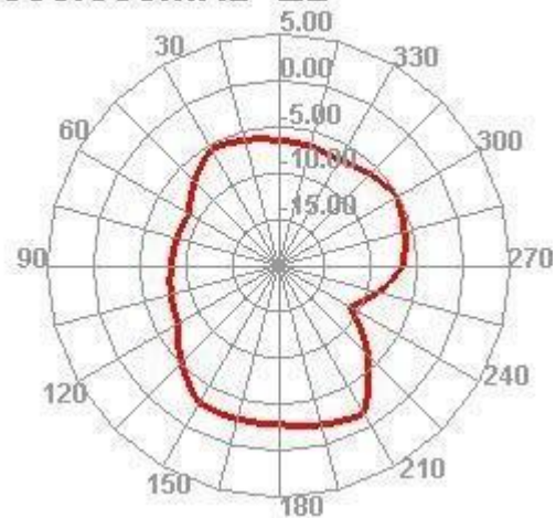
850.000MHz E2
