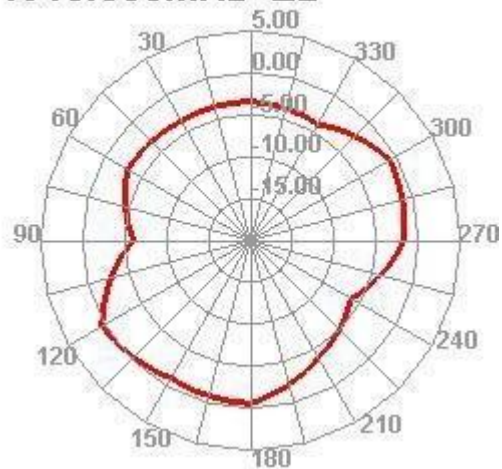
1910.000MHz E2
