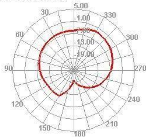
850.000MHz H
