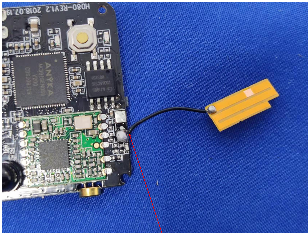
FPC natenna
