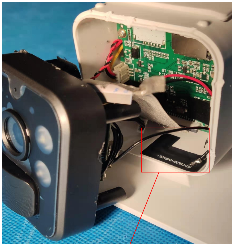
Antenna
