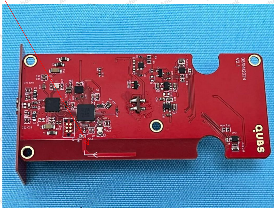
BLE ANT
