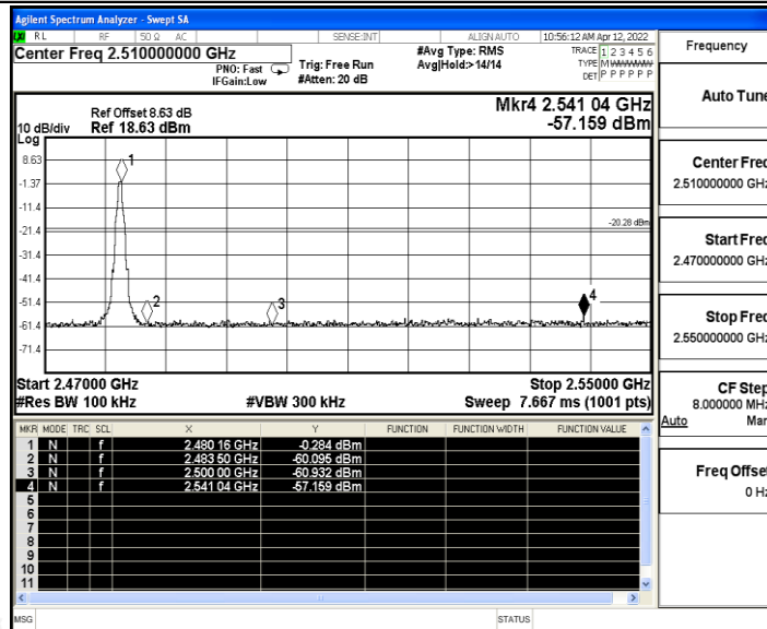
DH5_Ant_Low_Hop_2402
