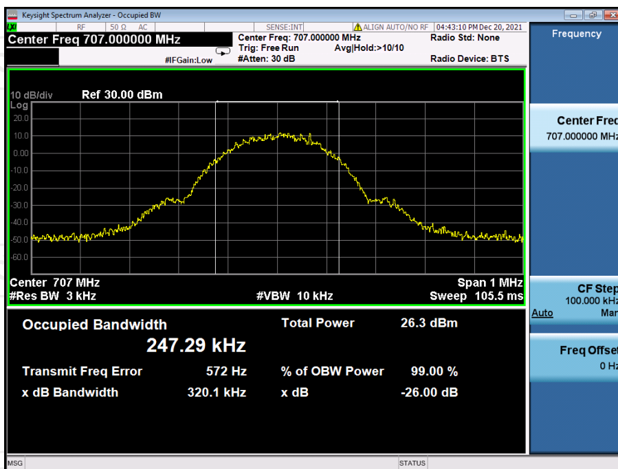
Lower700MHz GSM UL output
