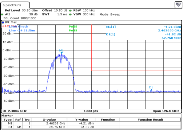
b_2462MHz_Chain 0
