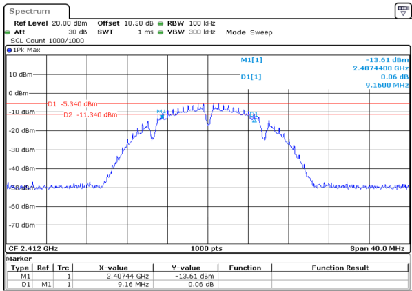
b_2412MHz_Chain 0 9.160MHz
