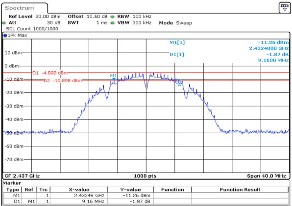
b_2437MHz_Chain 0 9.160MHz
