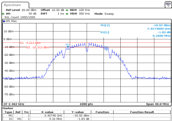
b_2462MHz_Chain 0 9.160MHz
