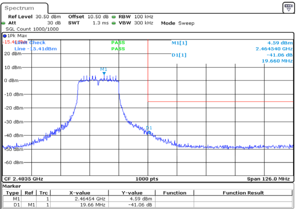
n20_2462MHz_Chain 0
