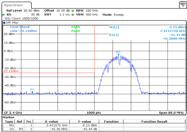
b_2412MHz_Chain 0
