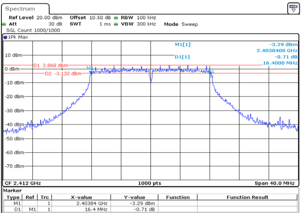
g_2412MHz_Chain 0 16.400MHz
