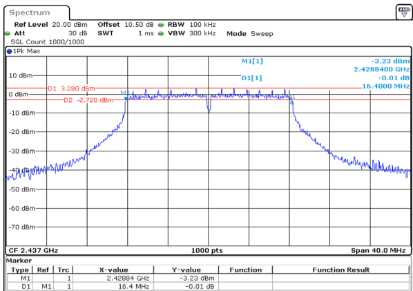
g_2437MHz_Chain 0 16.400MHz
