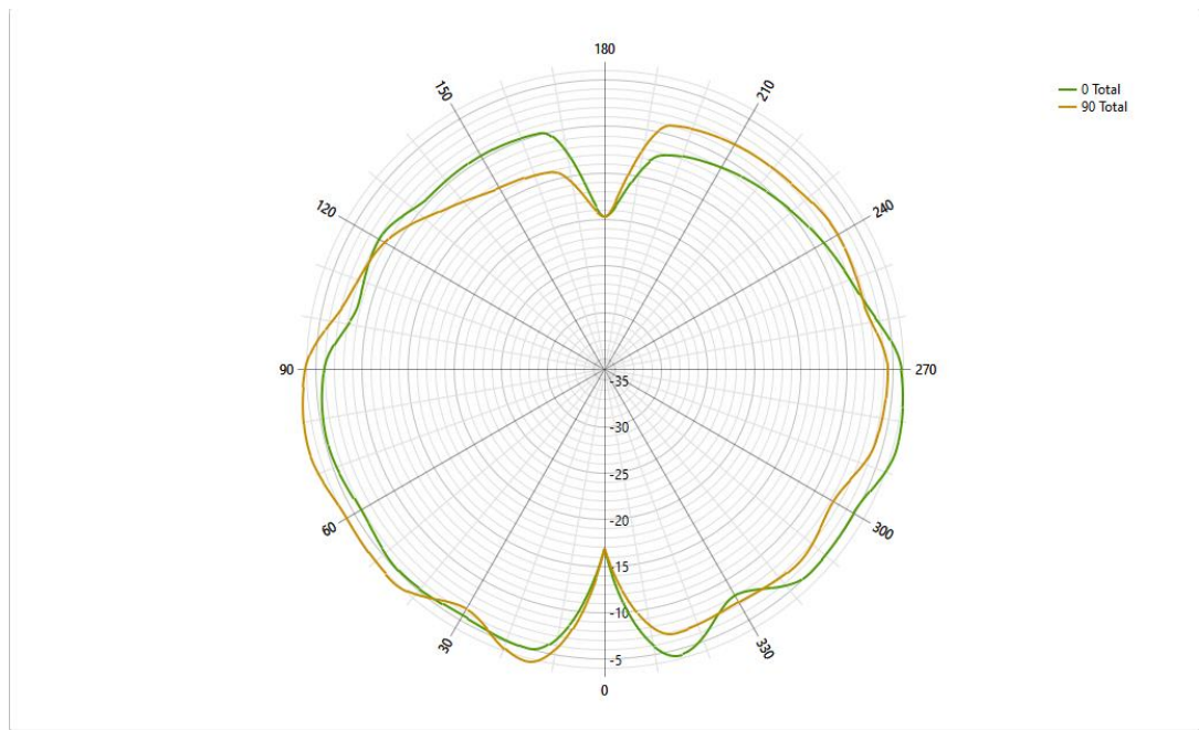
Phi=0 & Phi=90 °_2500MHz
