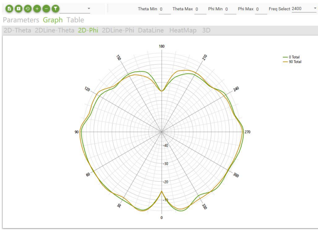
Phi=0 °&Phi=90 °_2400MHz
