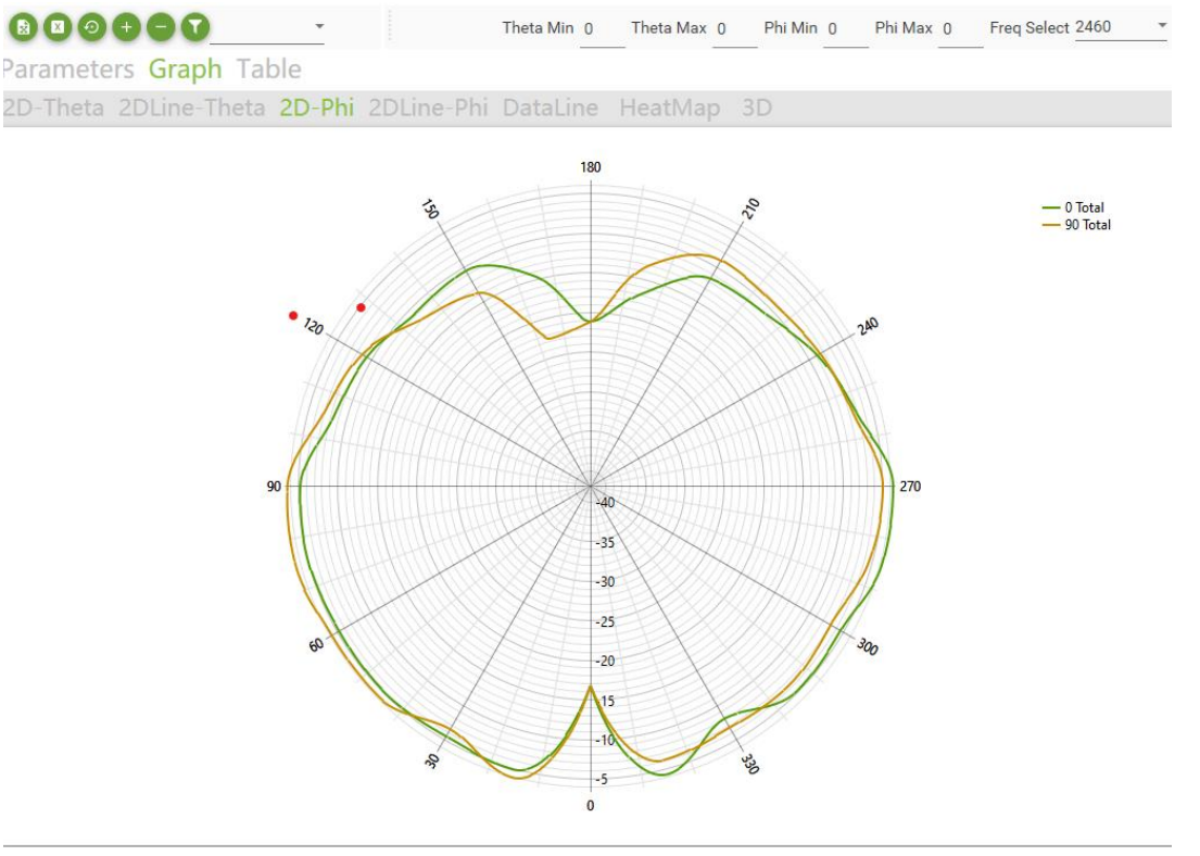
Phi=0 °&Phi=90 °_2460MHz
