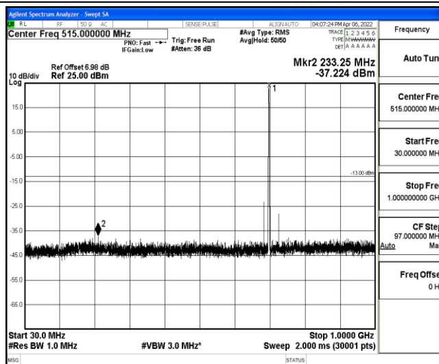
Band12-5MHz-16QAM-23095-1-0-Low-30-1000--37.22-PASS
