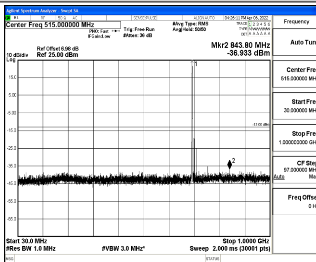
Band12-10MHz-QPSK-23060-1-0-Low-30-1000--36.93-PASS
