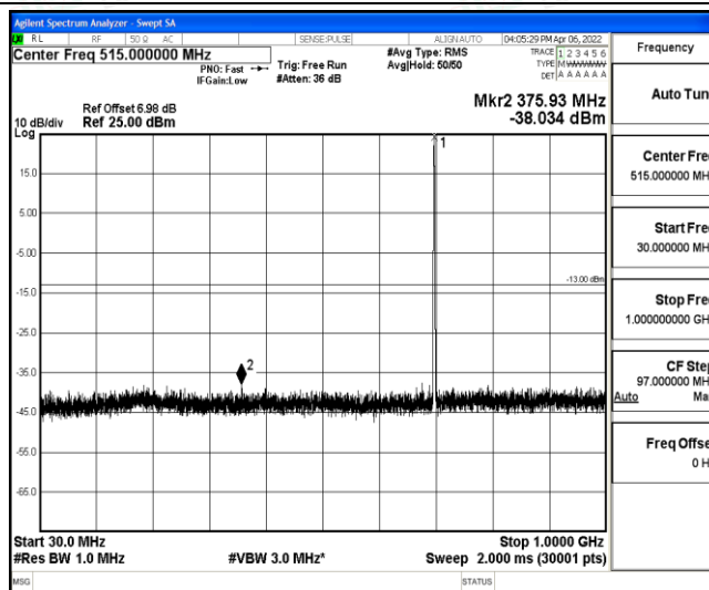
Band12-5MHz-QPSK-23095-1-0-Low-30-1000--38.03-PASS
