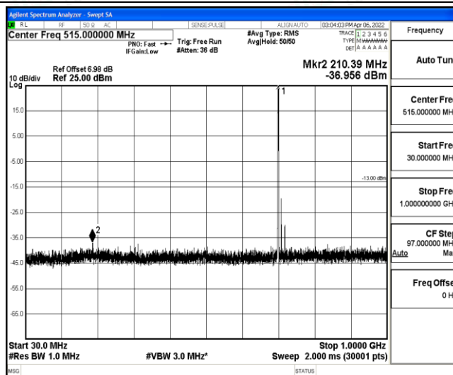
Band12-1.4MHz-QPSK-23095-1-0-Low-30-1000--36.96-PASS
