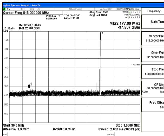
Band12-3MHz-QPSK-23095-1-0-Low-30-1000--37.81-PASS
