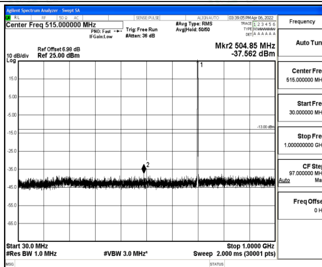
Band12-3MHz-16QAM-23095-1-0-Low-30-1000--37.56-PASS
