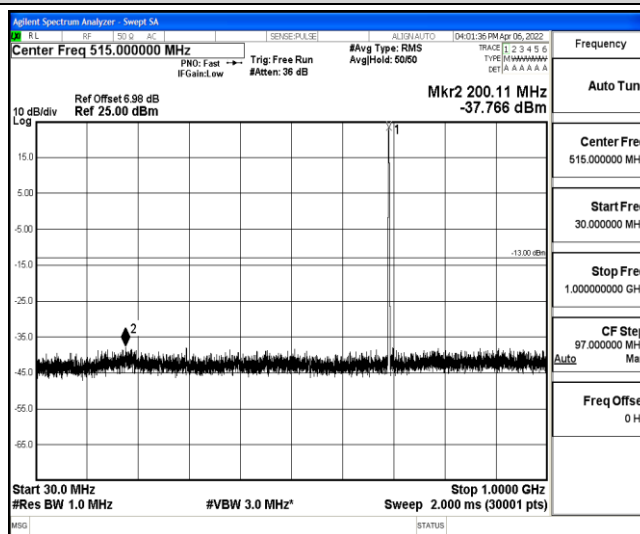
Band12-5MHz-QPSK-23035-1-0-Low-30-1000--37.77-PASS
