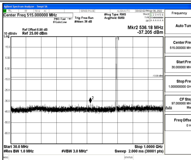
Band12-1.4MHz-16QAM-23017-1-0-Low-30-1000--37.21-PASS
