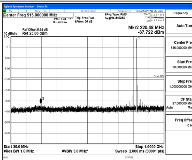
Band5-10MHz-QPSK-20450-1-0-Low-30-1000--37.72-PASS
