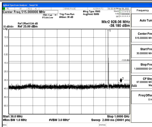
Band5-3MHz-QPSK-20415-1-0-Low-30-1000--38.18-PASS
