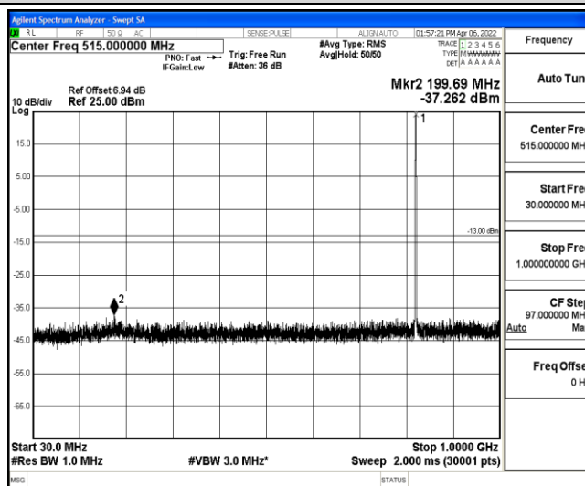
Band5-5MHz-QPSK-20425-1-0-Low-30-1000--37.26-PASS
