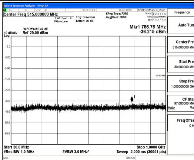
Band4-20MHz-QPSK-20050-1-0-Low-30-1000--36.22-PASS
