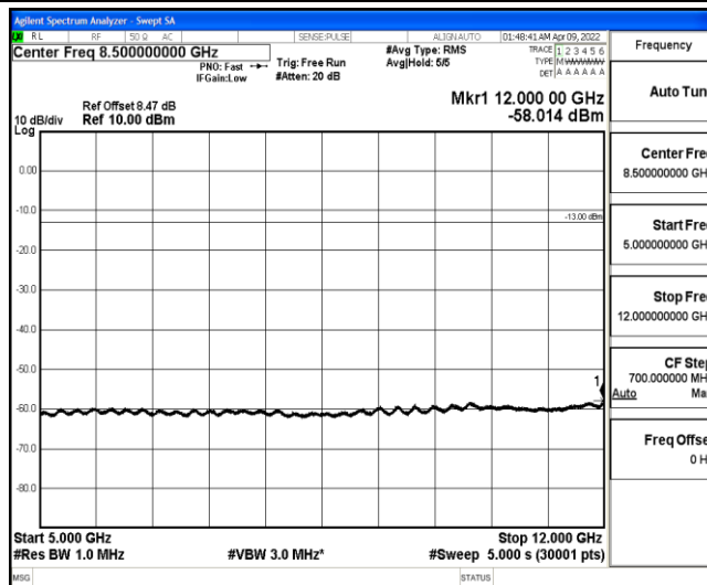
Band4-10MHz-QPSK-20175-1-0-Low-5000-12000--58.01-PASS
