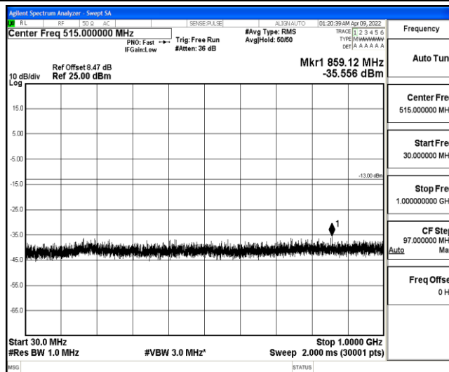
Band4-5MHz-QPSK-19975-1-0-Low-30-1000--35.56-PASS
