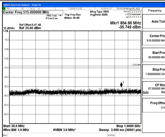
Band4-10MHz-QPSK-20000-1-0-Low-30-1000--35.75-PASS
