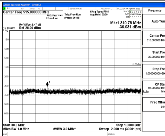
Band4-5MHz-16QAM-19975-1-0-Low-30-1000--36.03-PASS
