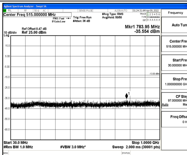
Band4-5MHz-QPSK-20175-1-0-Low-30-1000--35.55-PASS
