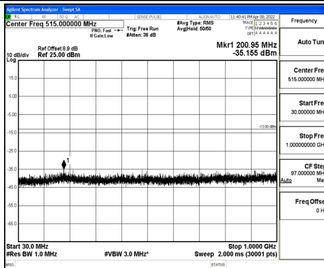
Band2-20MHz-QPSK-18700-1-0-Low-30-1000--35.16-PASS
