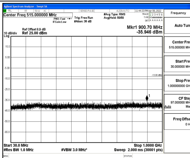
Band2-20MHz-QPSK-18900-1-0-Low-30-1000--35.95-PASS
