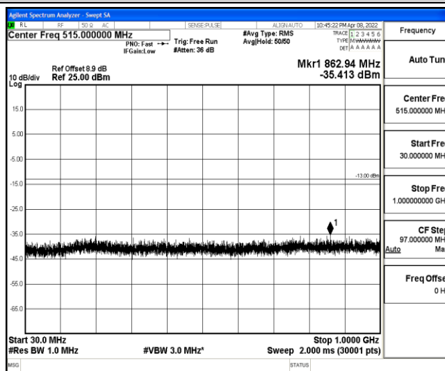
Band2-10MHz-QPSK-18900-1-0-Low-30-1000--35.41-PASS
