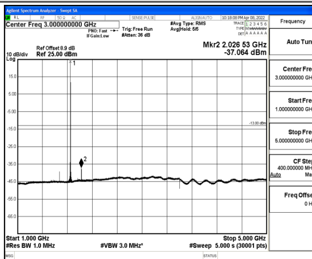
Band2-5MHz-QPSK-18625-1-0-Low-1000-5000--37.06-PASS
