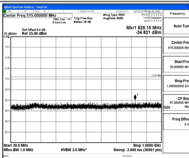
Band2-5MHz-QPSK-18900-1-0-Low-30-1000--34.82-PASS
