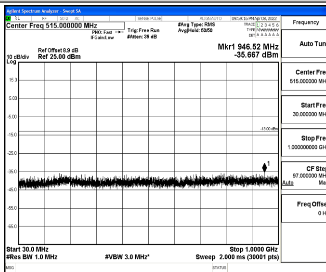
Band2-3MHz-16QAM-18900-1-0-Low-30-1000--35.67-PASS
