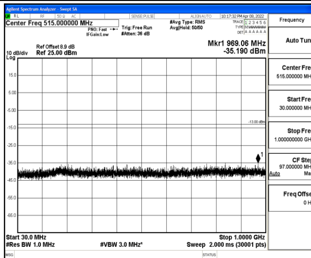
Band2-5MHz-QPSK-18625-1-0-Low-30-1000--35.19-PASS
