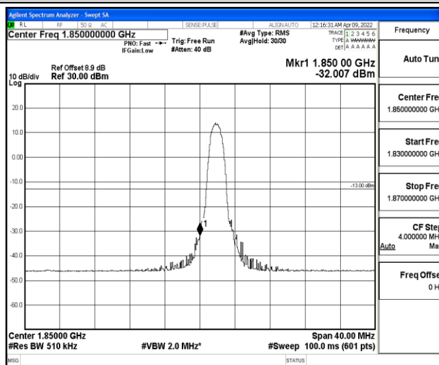
Band2-20MHz-16QAM-18700-6-0-Low--32.01-PASS
