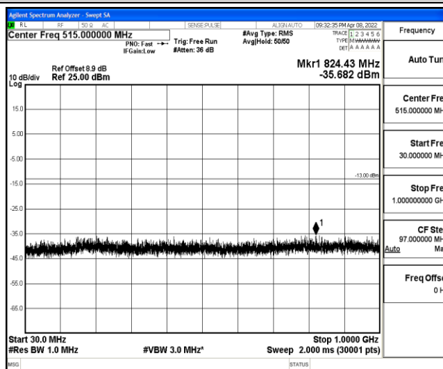
Band2-1.4MHz-QPSK-18900-1-0-Low-30-1000--35.68-PASS
