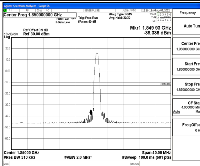
Band2-20MHz-16QAM-18700-1-0-Low--39.34-PASS
