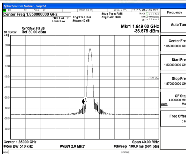
Band2-20MHz-QPSK-18700-1-0-Low--36.57-PASS
