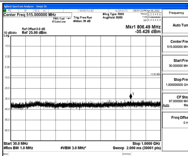
Band2-3MHz-QPSK-18900-1-0-Low-30-1000--35.43-PASS
