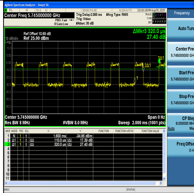
NTNV-11AX20MIMO-Ant1-5745
