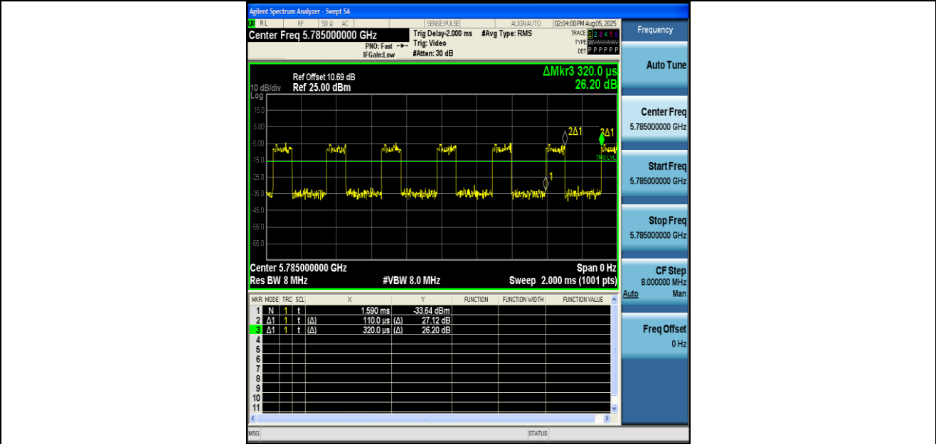
NTNV-11AX20MIMO-Ant1-5785
