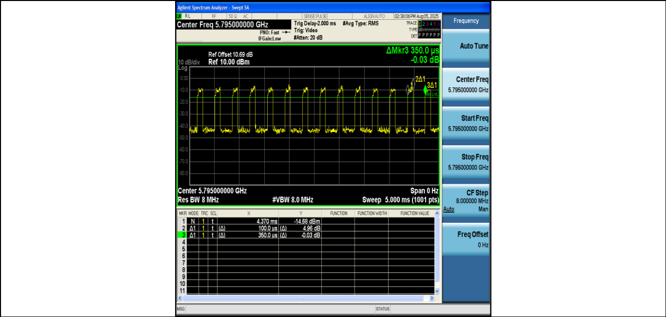
NTNV-11AX40MIMO-Ant2-5795
