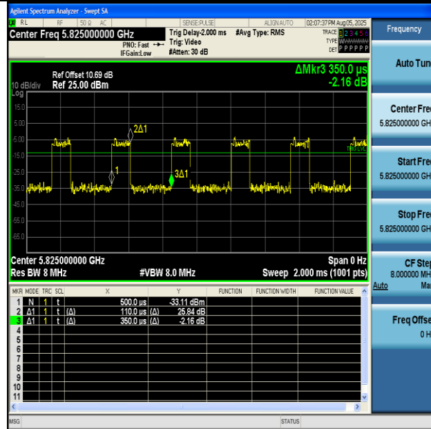
NTNV-11AX20MIMO-Ant1-5825
