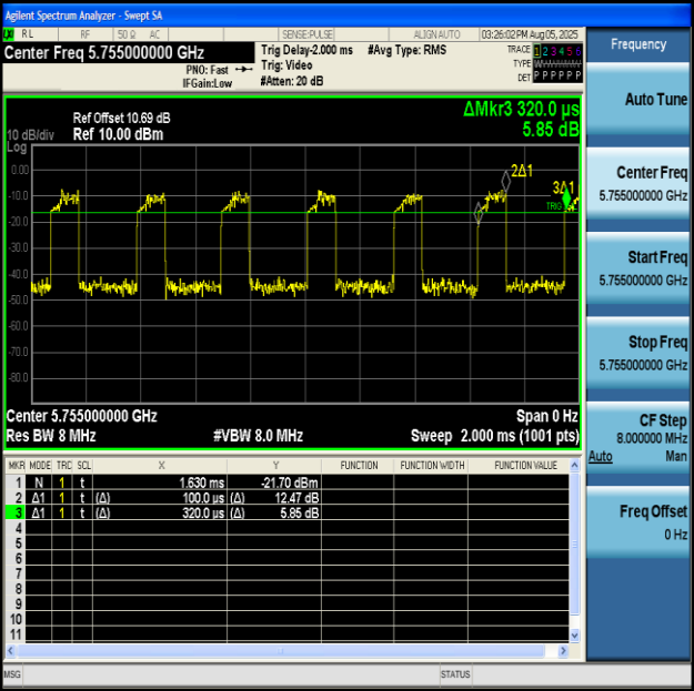
NTNV-11N40MIMO-Ant1-5755
