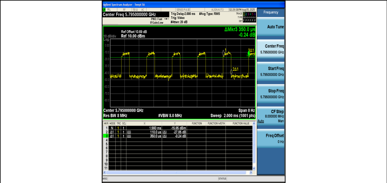
NTNV-11AX40MIMO-Ant1-5795
