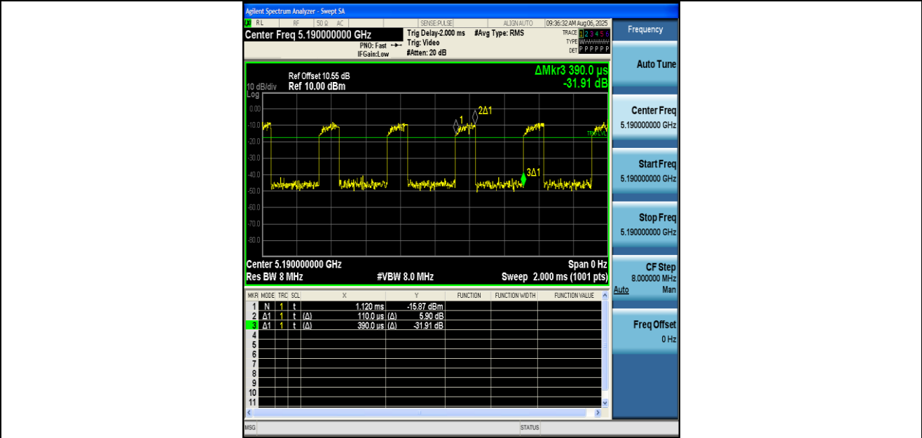
NTNV-11AX40MIMO-Ant1-5190
