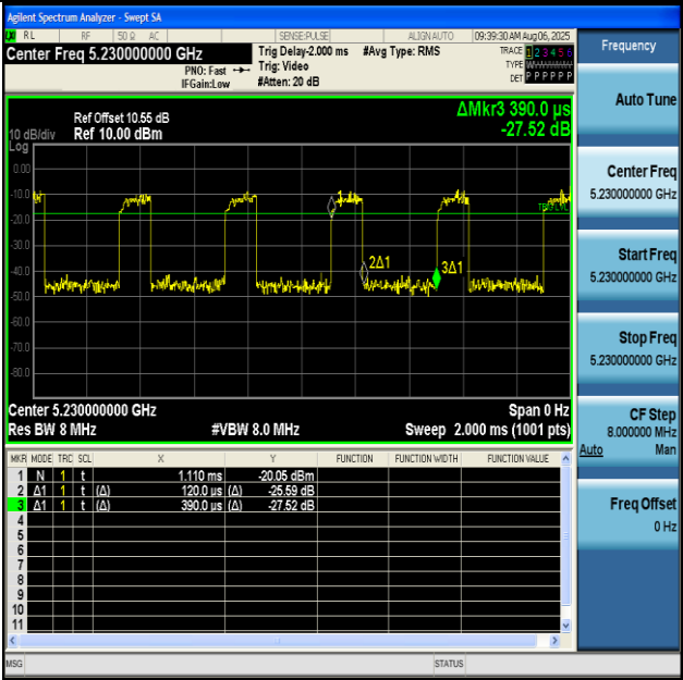
NTNV-11AX40MIMO-Ant1-5230
