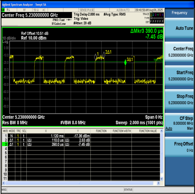
NTNV-11AX40MIMO-Ant2-5230
