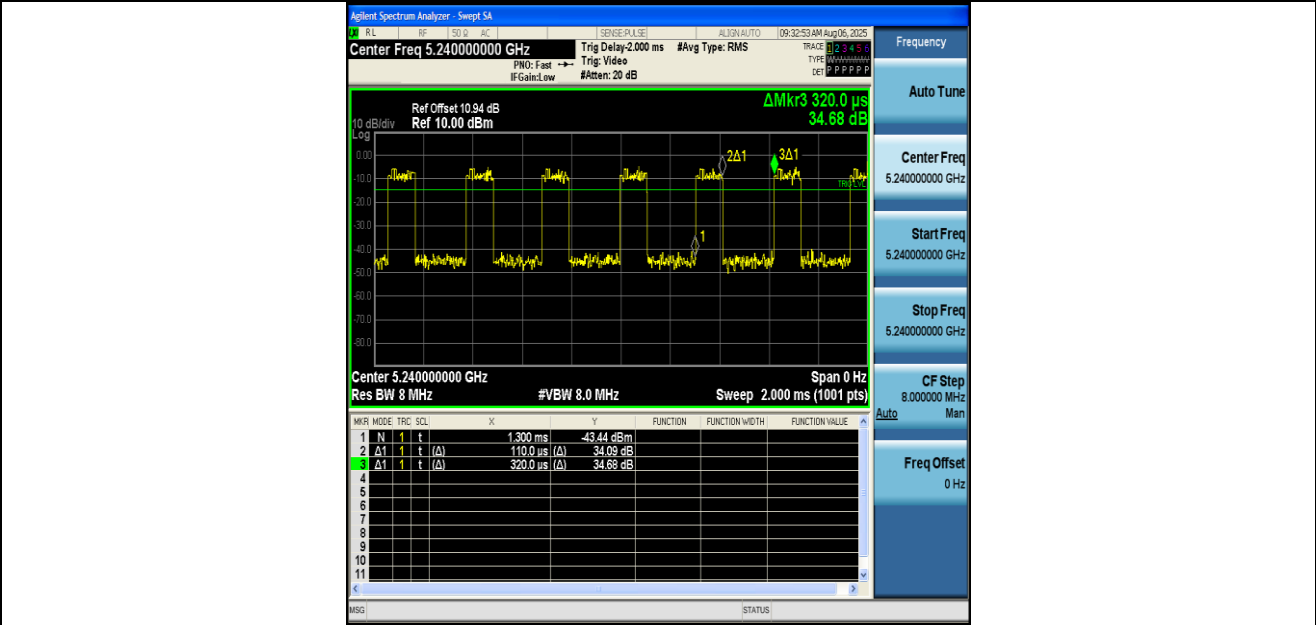
NTNV-11AX20MIMO-Ant1-5240
