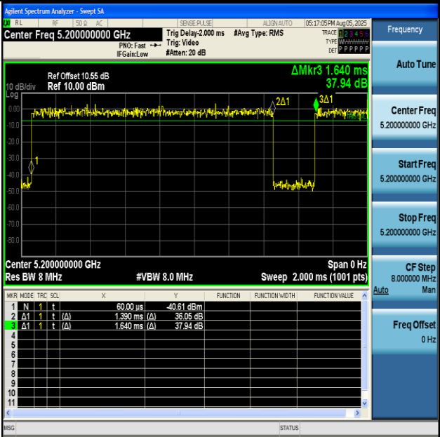
NTNV-11A-Ant1-5200
