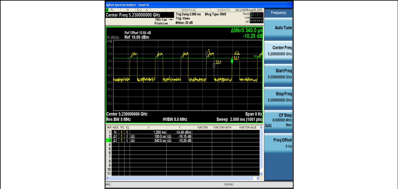
NTNV-11N40MIMO-Ant1-5230
