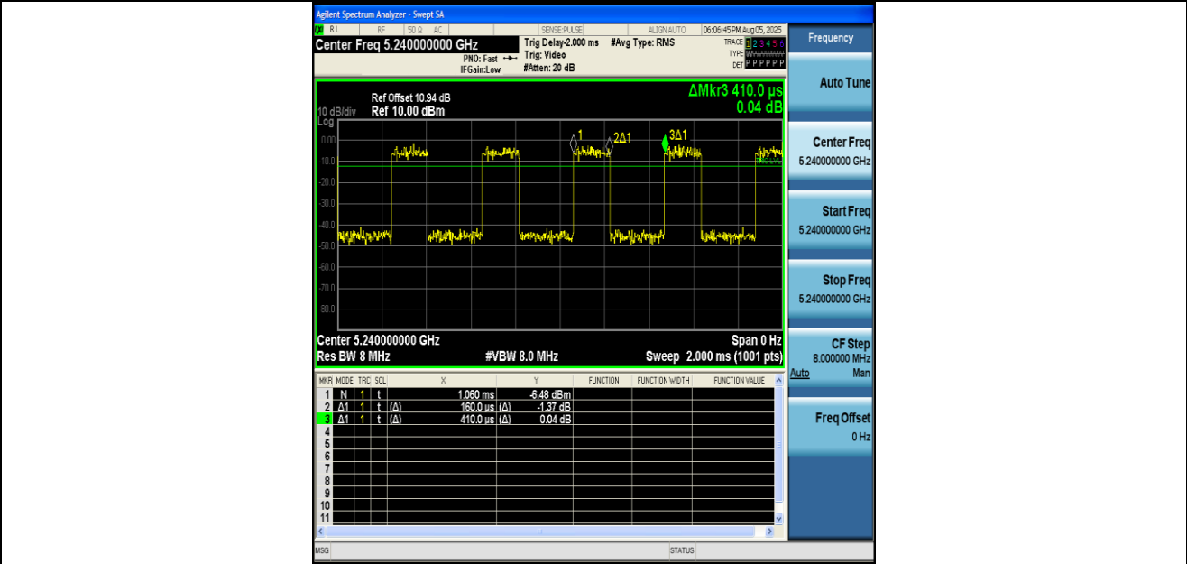
NTNV-11N20MIMO-Ant1-5240
