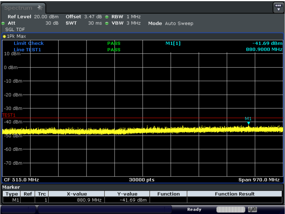
Test_Graph_11ax40_ANT1_6845_HE0_TX1
