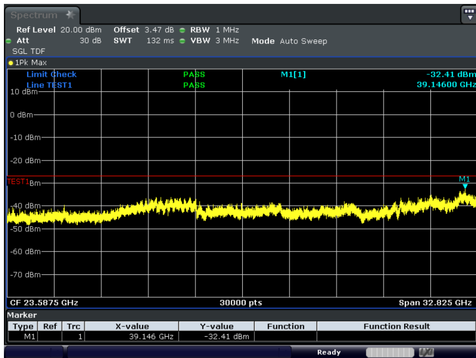
Test_Graph_11ax80_ANT1_5985_HE0_TX2
