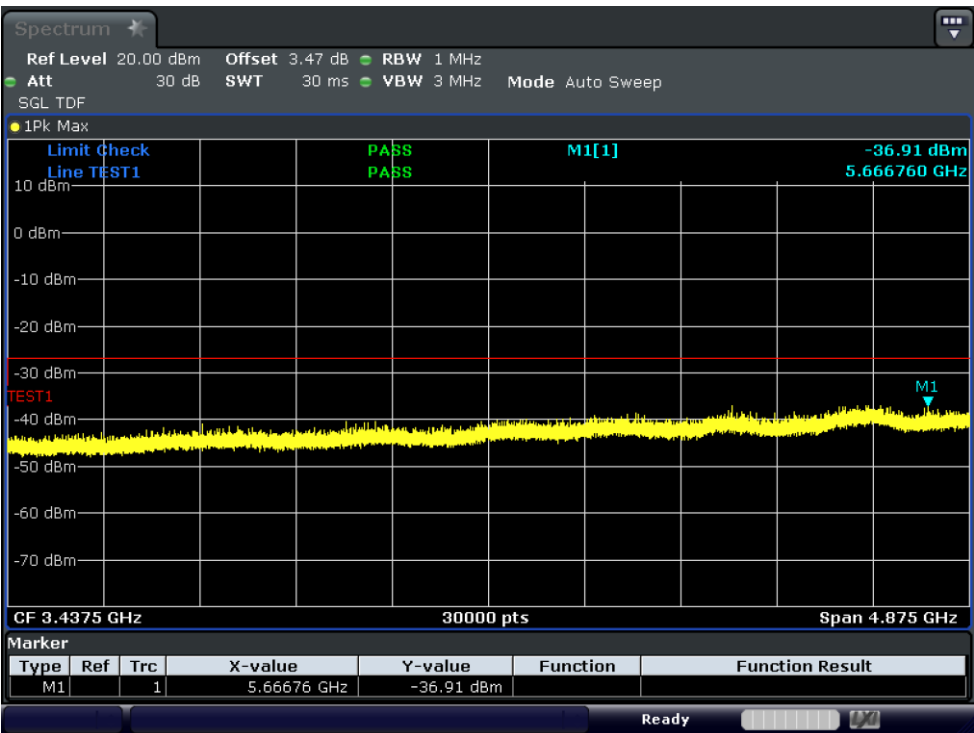
Test_Graph_11ax80_ANT1_6785_HE0_TX1
