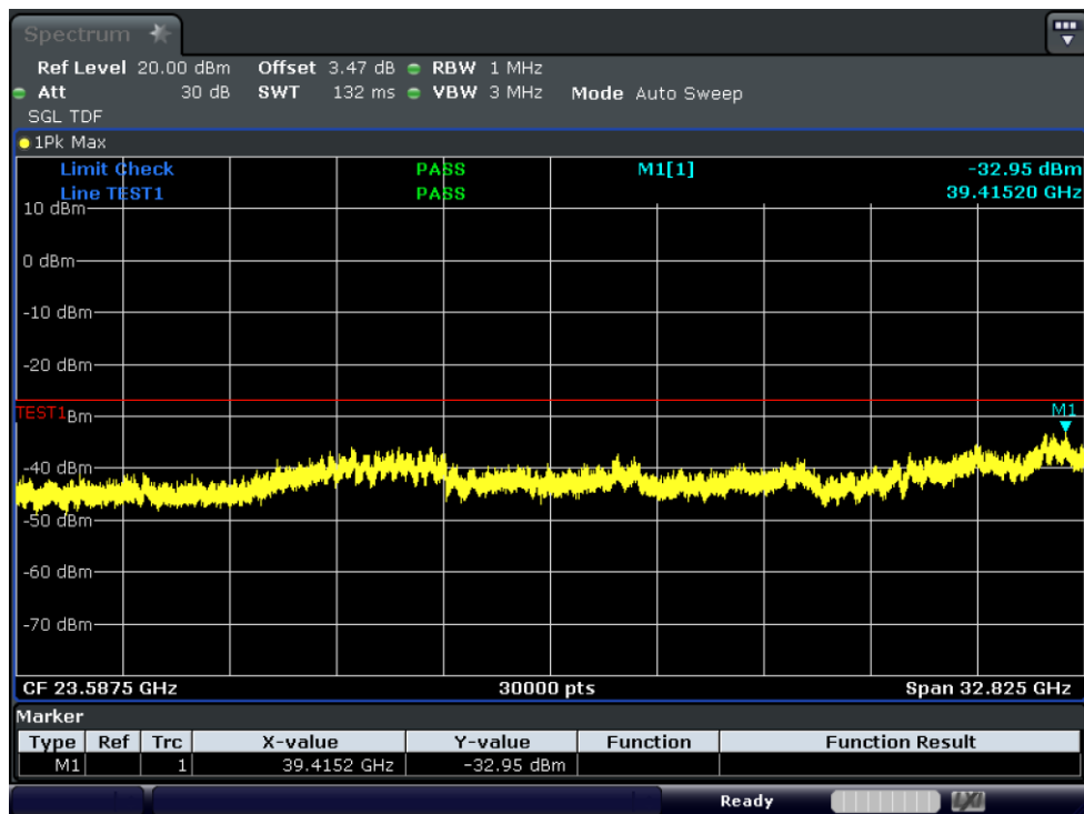
Test_Graph_11ax80_ANT1_6865_HE0_TX2
