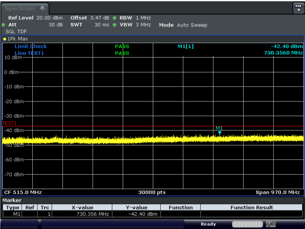
Test_Graph_11ax20_ANT1_6875_HE0_TX1
