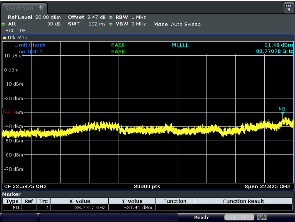
Test_Graph_11ax40_ANT1_6885_HE0_TX2
