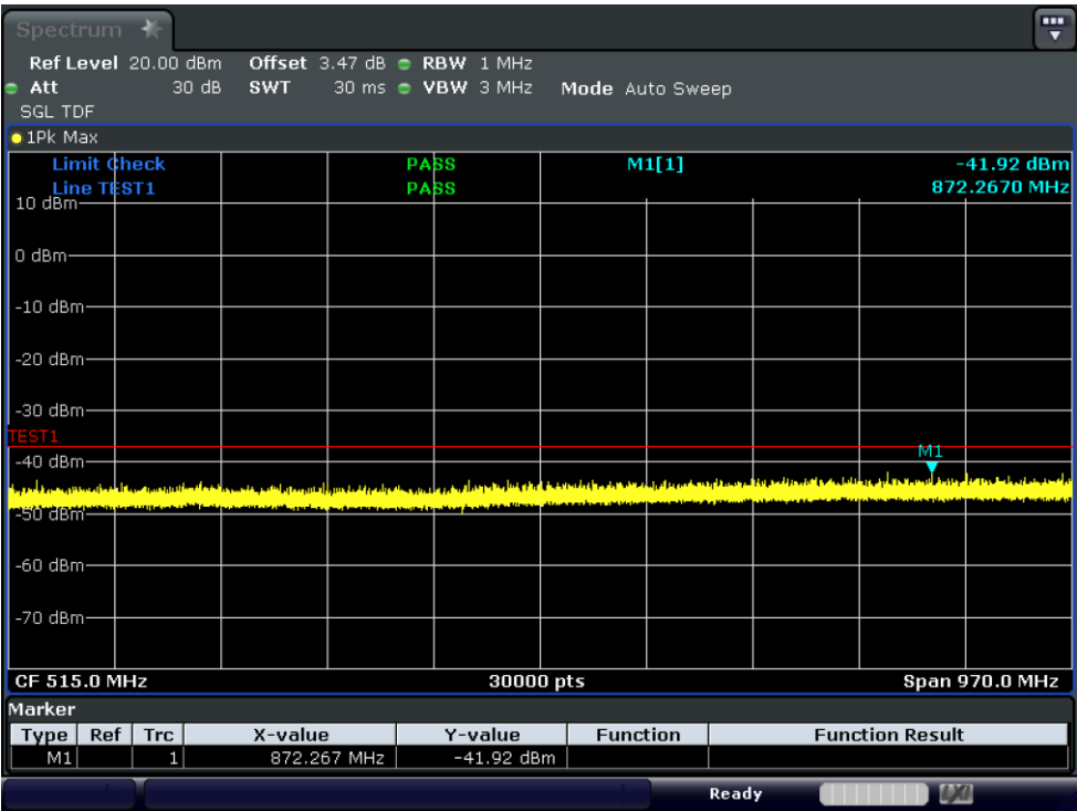
Test_Graph_11ax80_ANT1_6785_HE0_TX3
