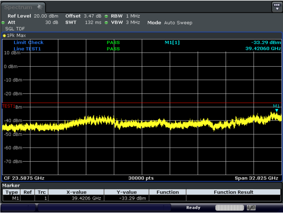
Test_Graph_11ax80_ANT1_6785_HE0_TX3
