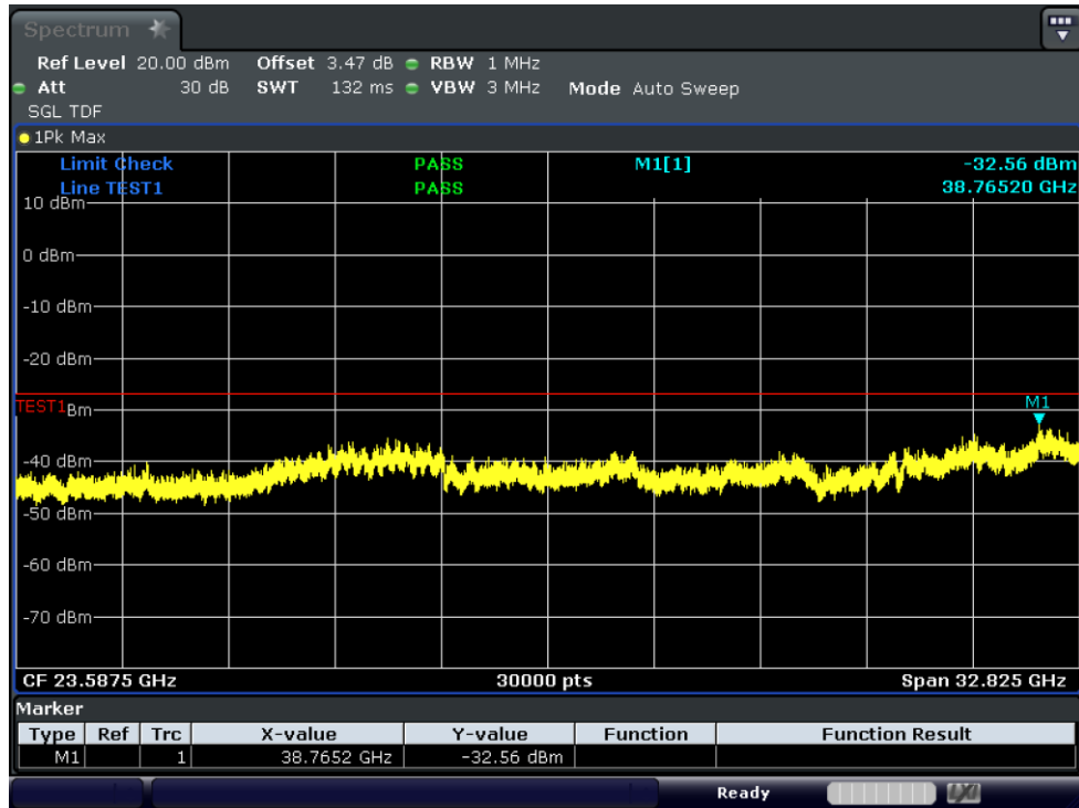
Test_Graph_11ax20_ANT1_6875_HE0_TX3
