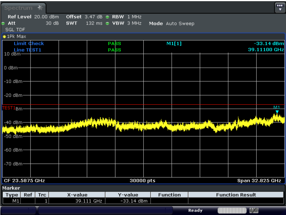
Test_Graph_11ax80_ANT1_6385_HE0_TX3
