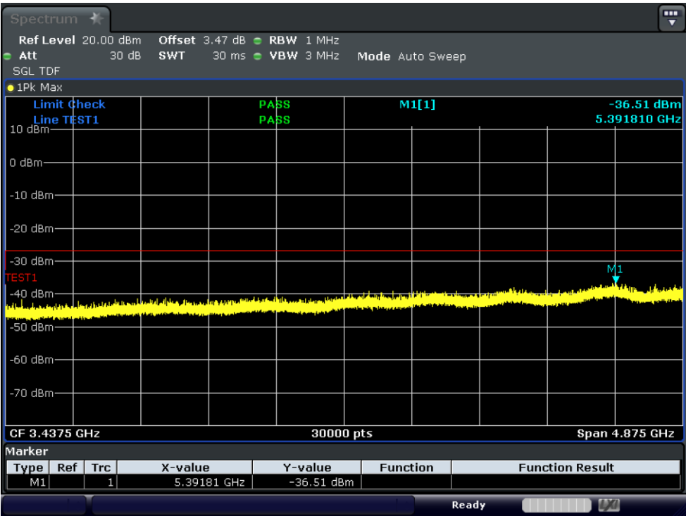
Test_Graph_11ax40_ANT1_7085_HE0_TX1
