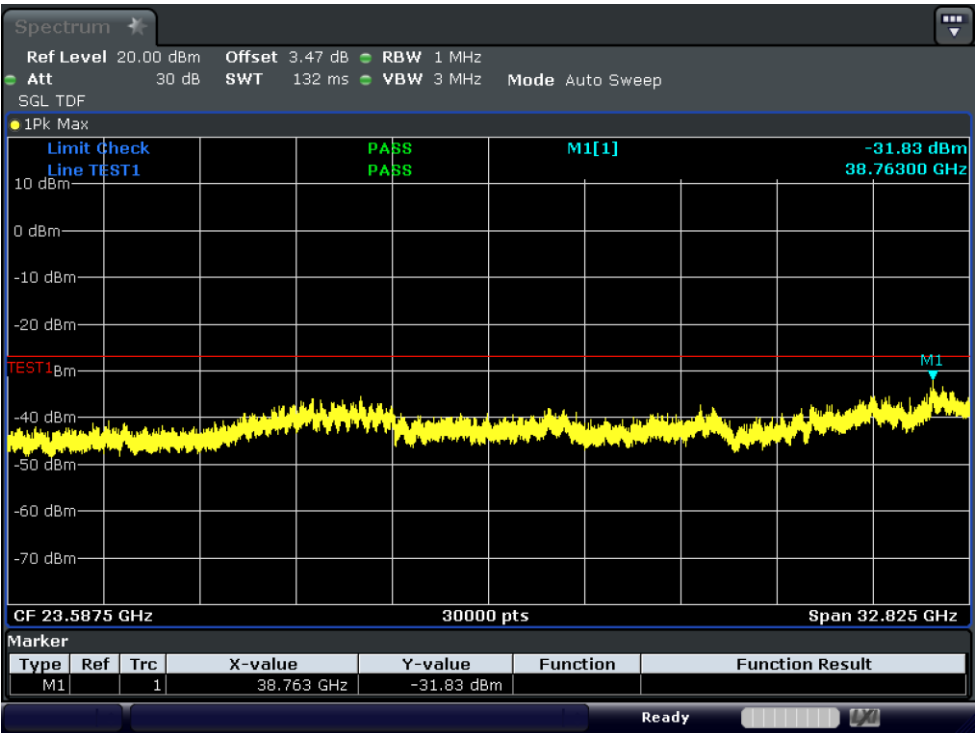
Test_Graph_11ax40_ANT1_6445_HE0_TX3
