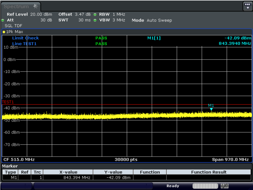
Test_Graph_11ax80_ANT1_6385_HE0_TX1
