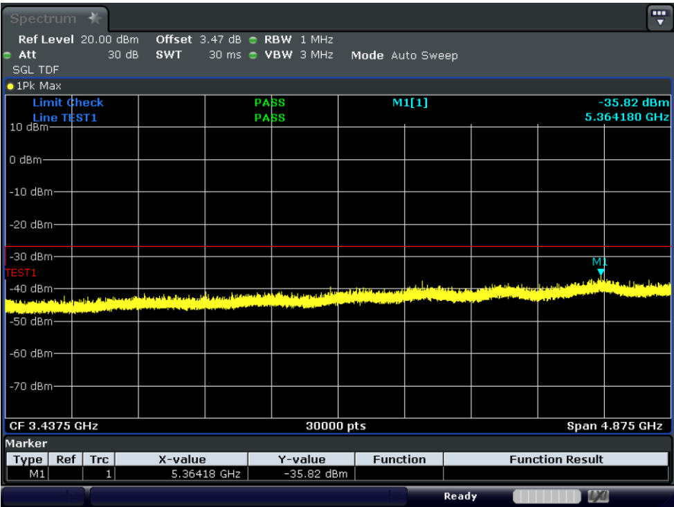
Test_Graph_11ax20_ANT1_6535_HE0_TX1
