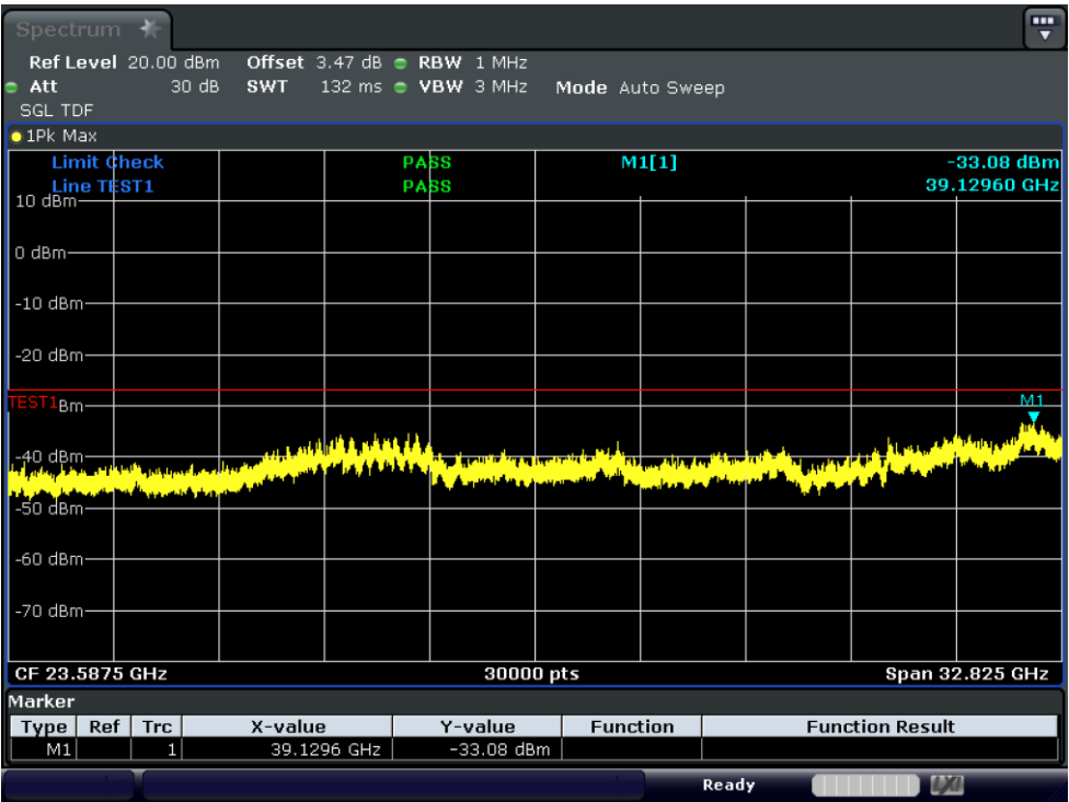
Test_Graph_11ax40_ANT1_6845_HE0_TX3
