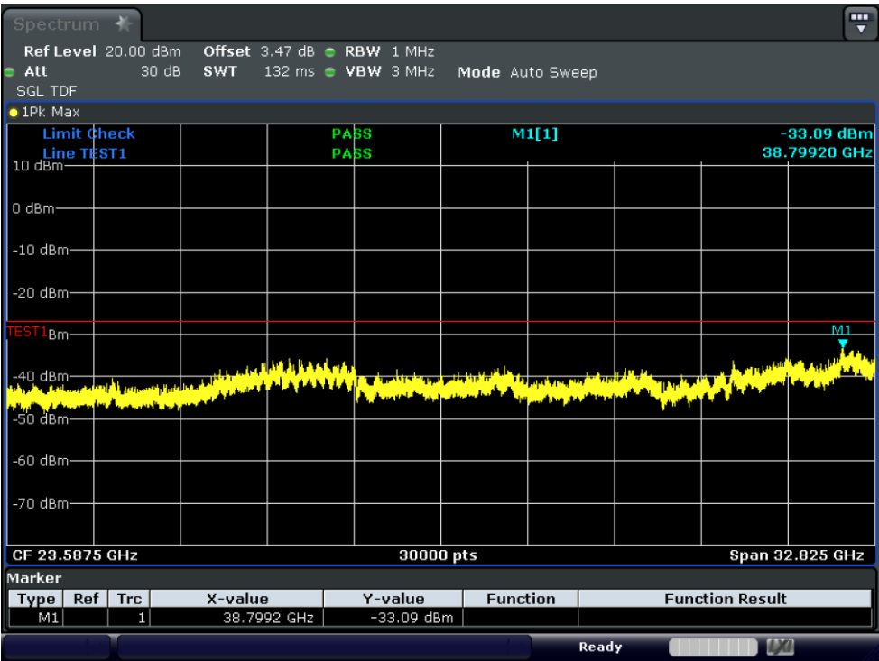
Test_Graph_11ax20_ANT1_7115_HE0_TX2
