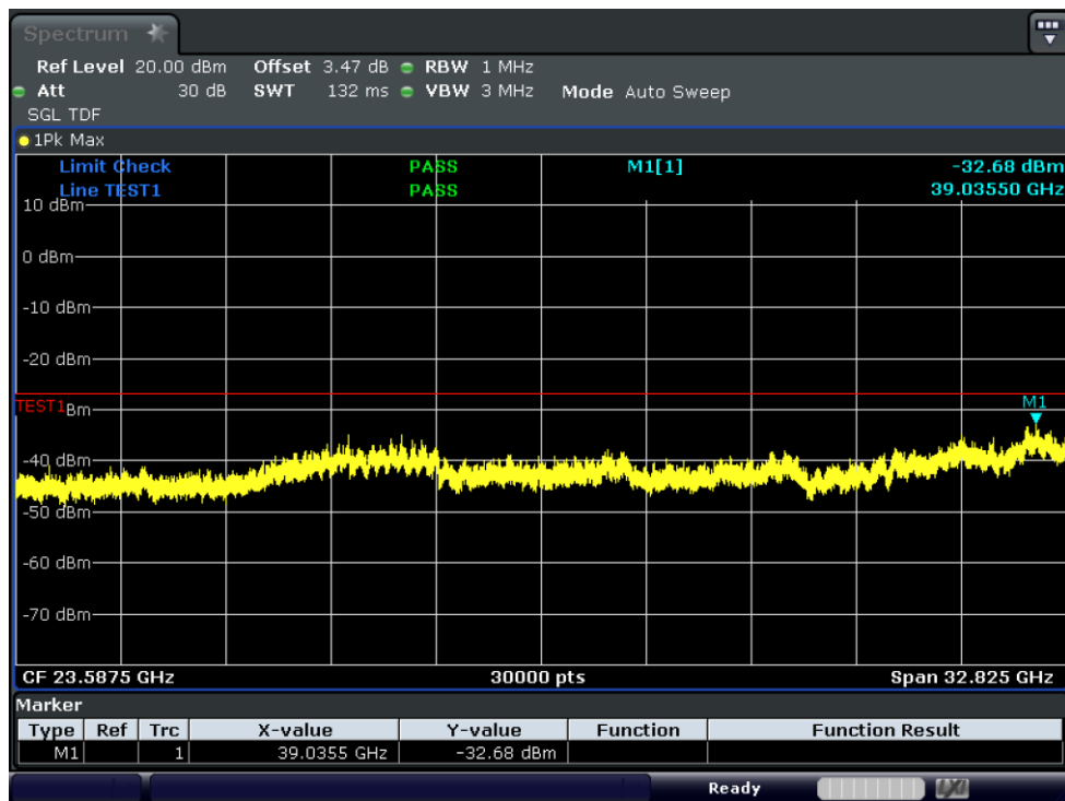
Test_Graph_11ax40_ANT1_6405_HE0_TX2
