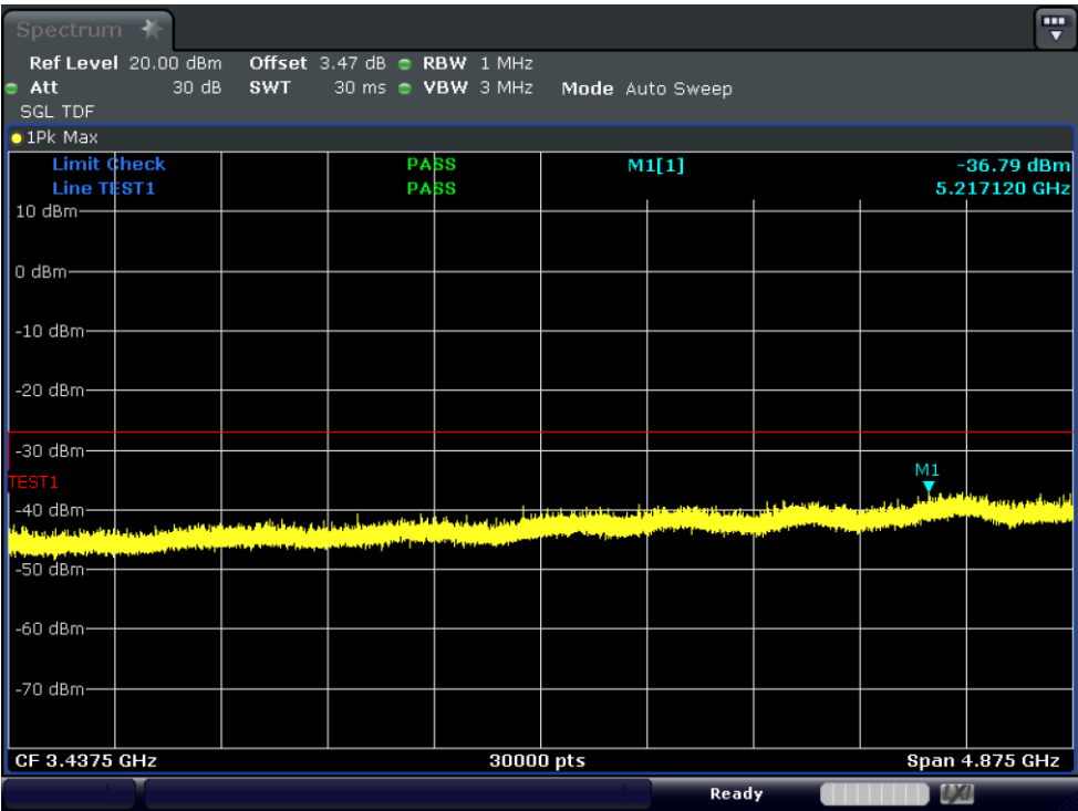
Test_Graph_11ax20_ANT1_6515_HE0_TX2
