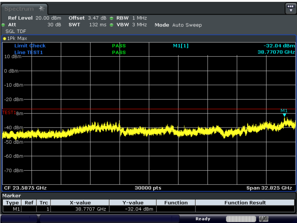
Test_Graph_11ax40_ANT1_6525_HE0_TX2
