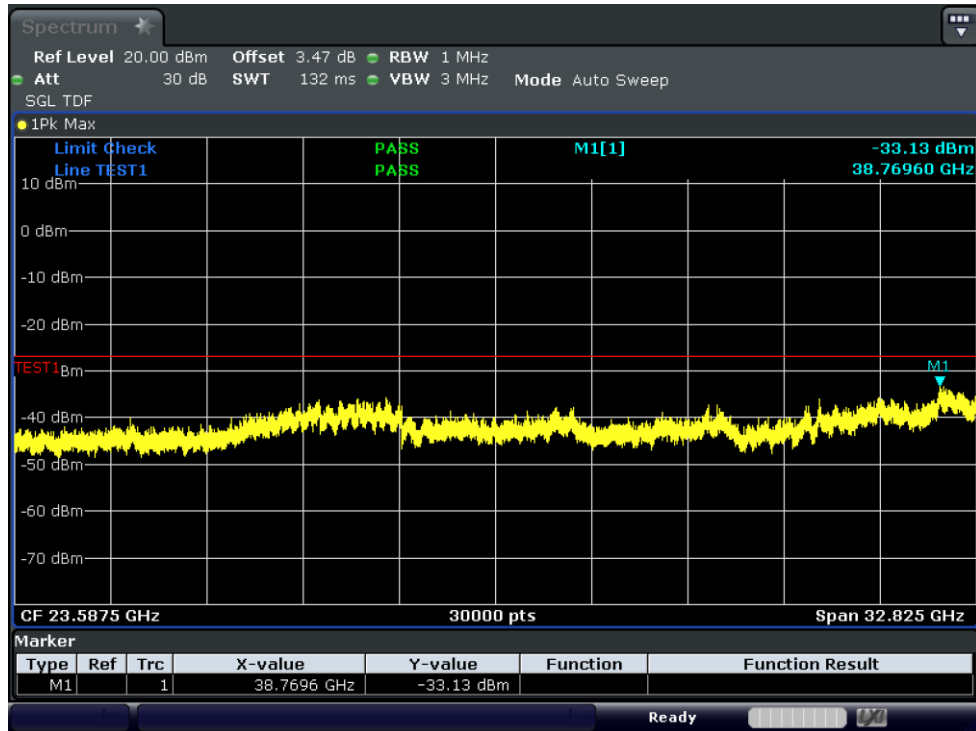
Test_Graph_11ax80_ANT1_6545_HE0_TX3
