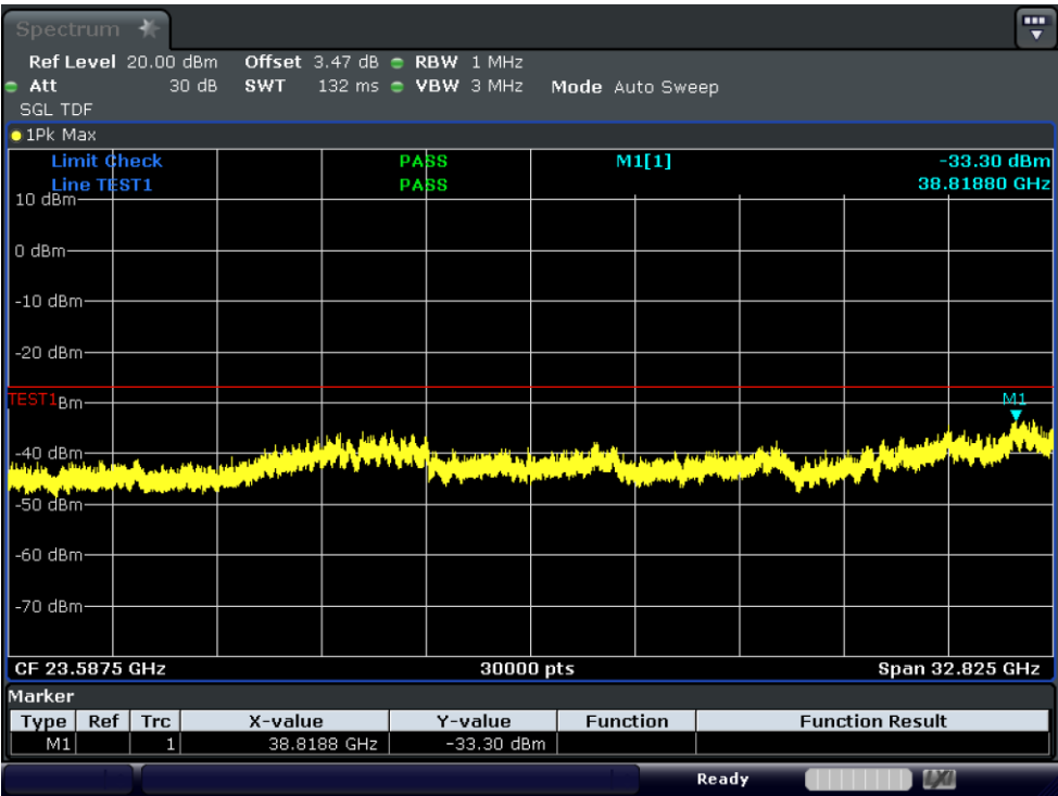
Test_Graph_11ax20_ANT1_6535_HE0_TX3
