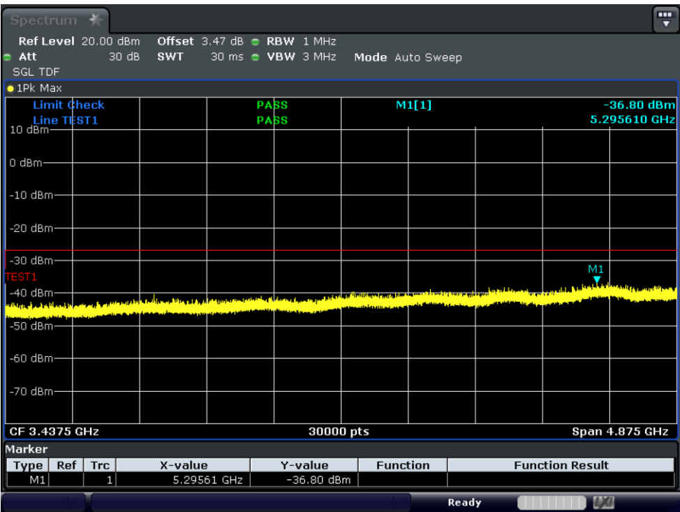
Test_Graph_11ax80_ANT1_6545_HE0_TX1
