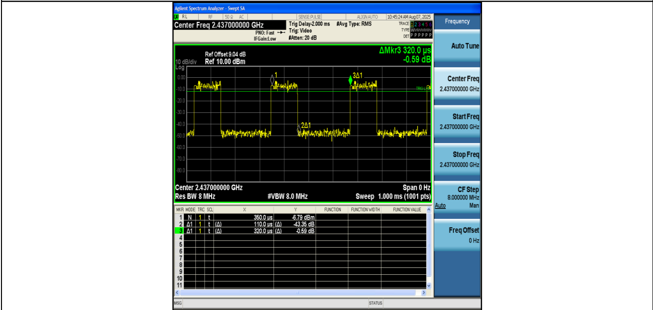
NTNV-11AX20MIMO-Ant2-2437
