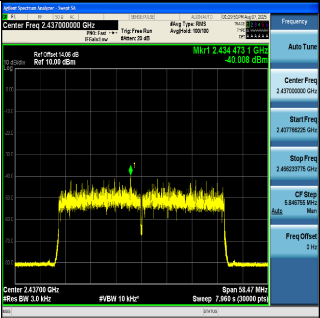
11AX40MIMO-Ant1-2437-PASS
