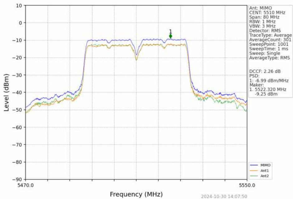
802.11n(HT40) LCH_5510MHz_MIMO_NTNV
