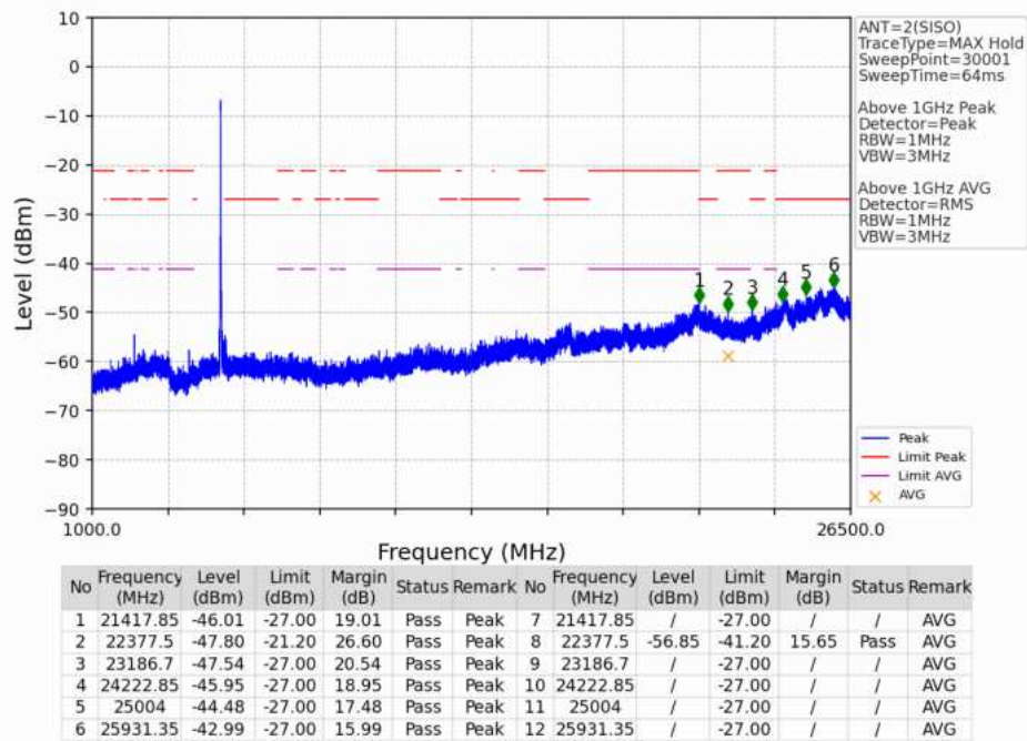
802.11a_HCH_5320MHz_Ant2_NTNV
