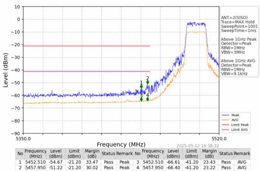
802.11a_LCH_5500MHz_Ant2_NTNV
