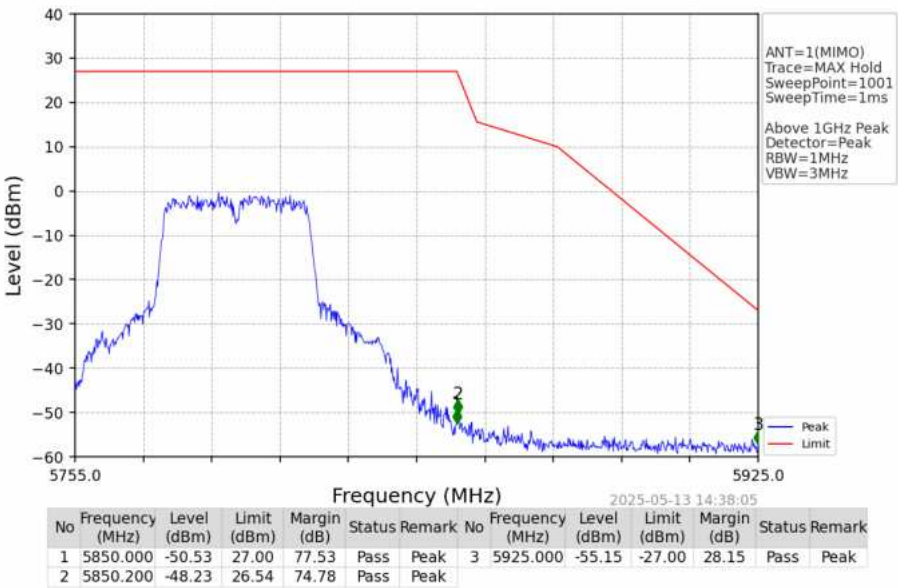
802.11n(HT40)_HCH_5795MHz_Ant1_NTNV
