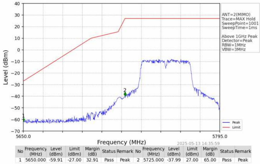
802.11n(HT40)_LCH_5755MHz_Ant2_NTNV
