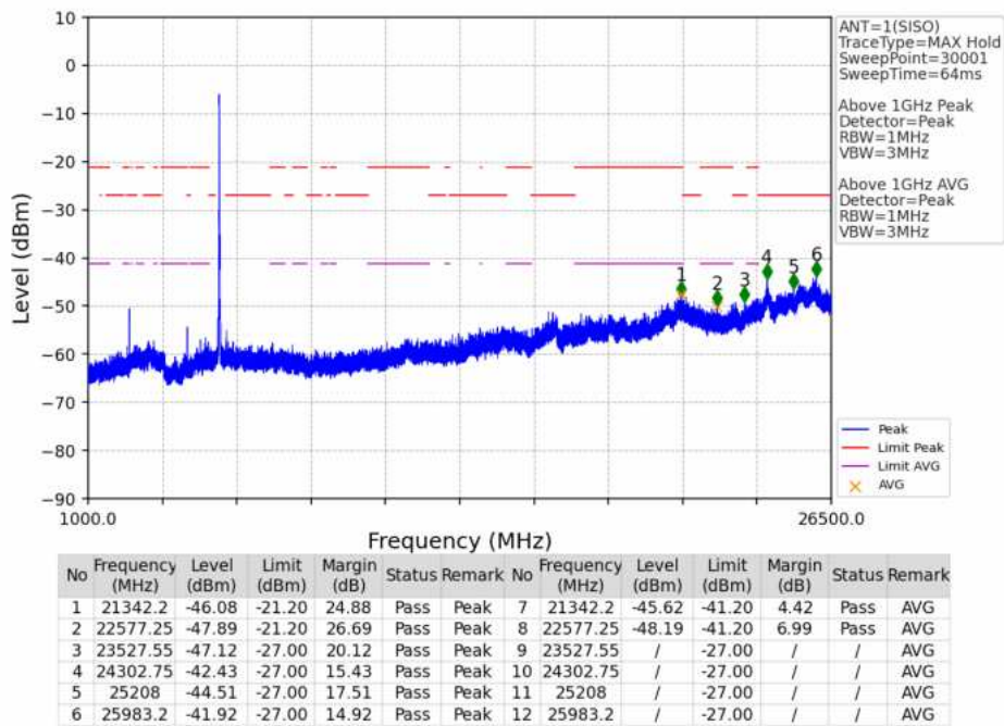
802.11a_LCH_5500MHz_Ant1_NTNV
