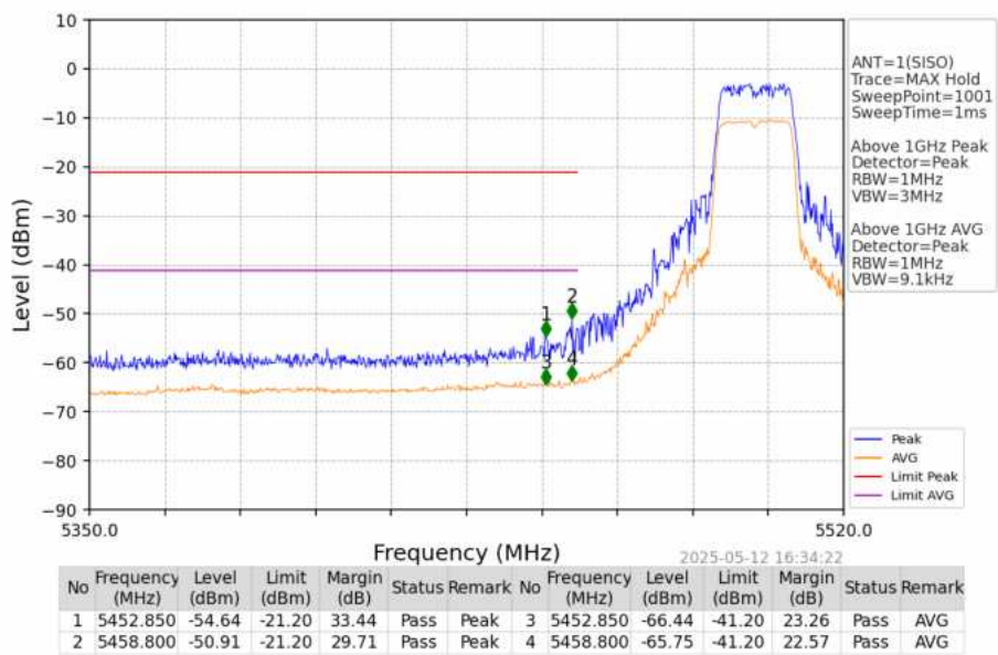
802.11a_LCH_5500MHz_Ant1_NTNV
