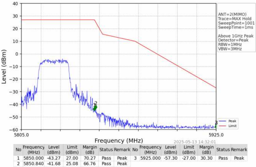
802.11n(HT20)_HCH_5825MHz_Ant2_NTNV
