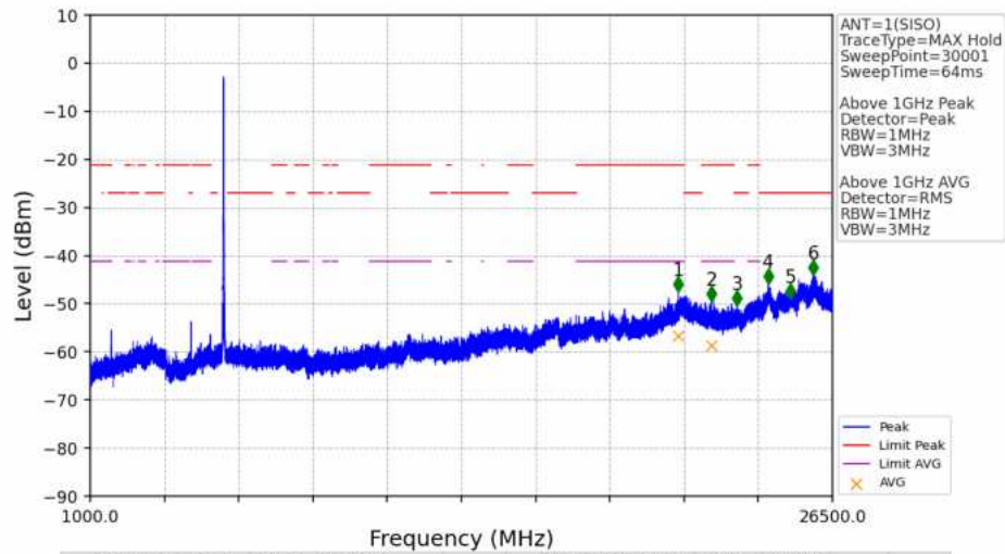
802.11a_MCH_5580MHz_Ant1_NTNV
