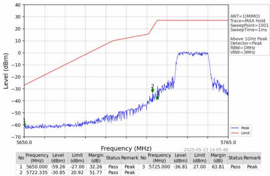
802.11n(HT20)_LCH_5745MHz_Ant1_NTNV
