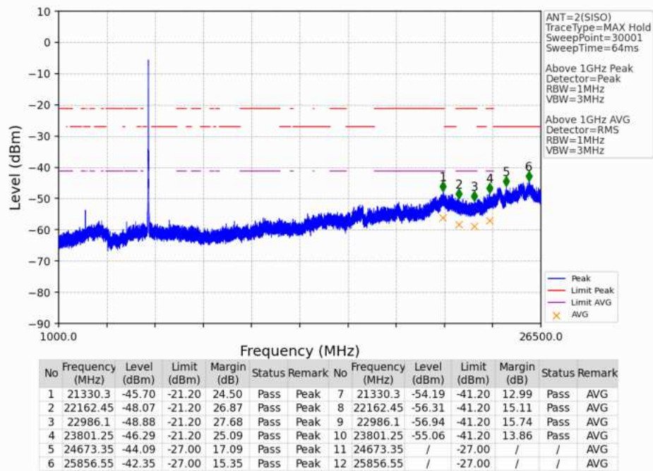
802.11a_LCH_5745MHz_Ant2_NTNV
