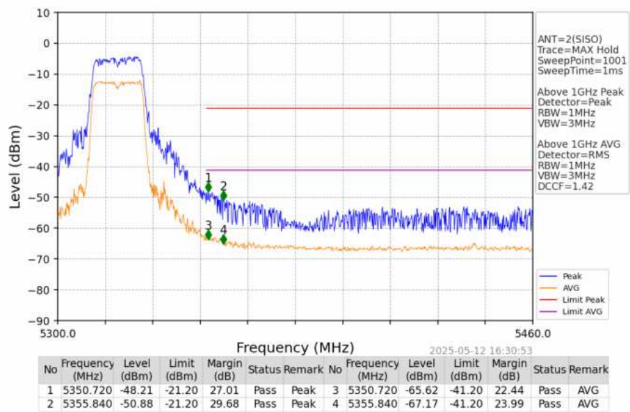
802.11a_HCH_5320MHz_Ant2_NTNV
