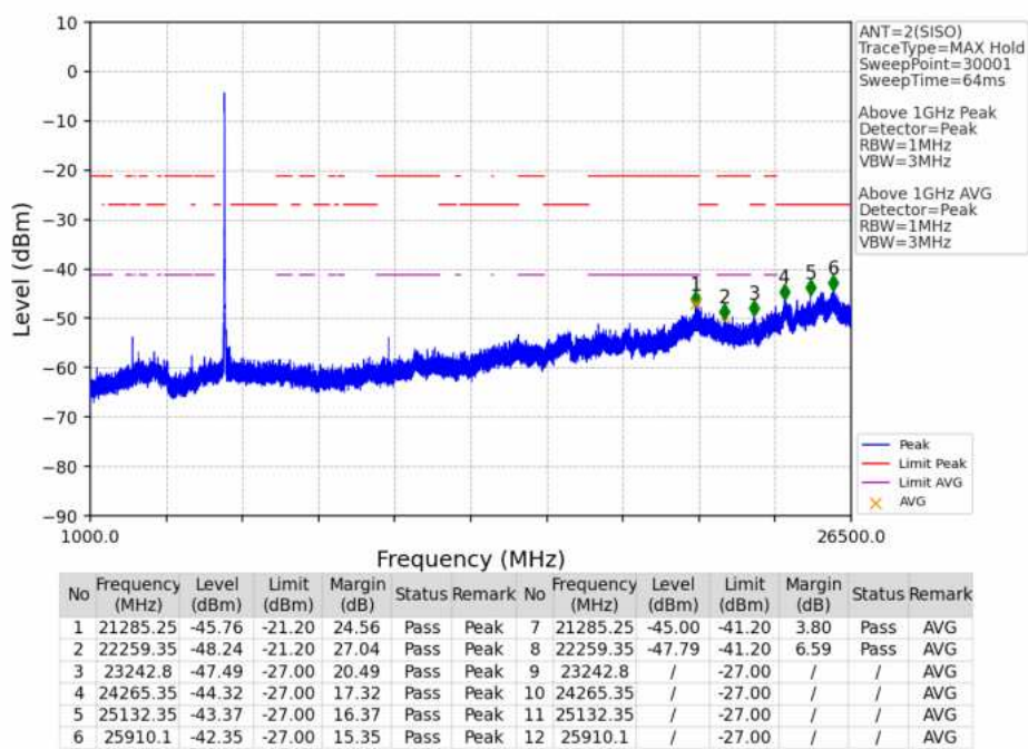
802.11a_LCH_5500MHz_Ant2_NTNV
