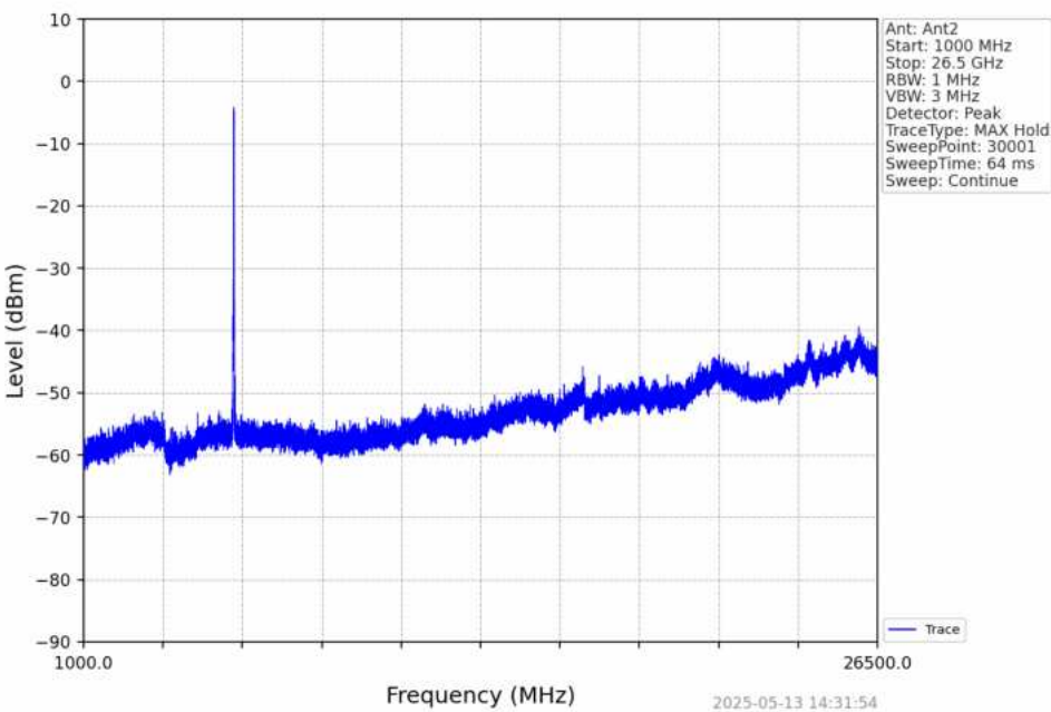
802.11n(HT20)_HCH_5825MHz_Ant2_NTNV
