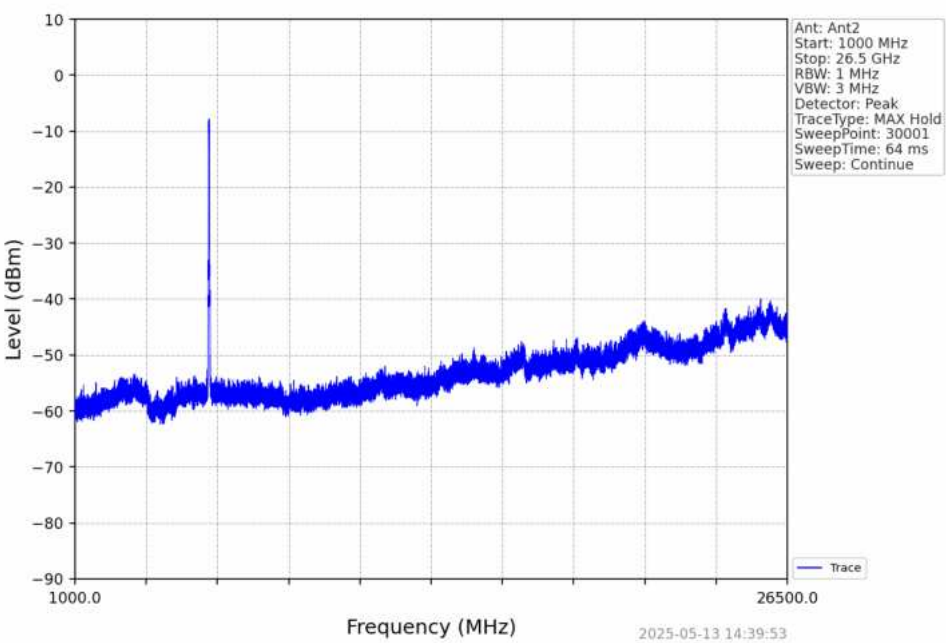
802.11n(HT40)_HCH_5795MHz_Ant2_NTNV
