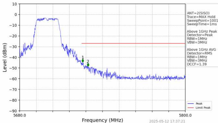
802.11a_HCH_5700MHz_Ant2_NTNV
