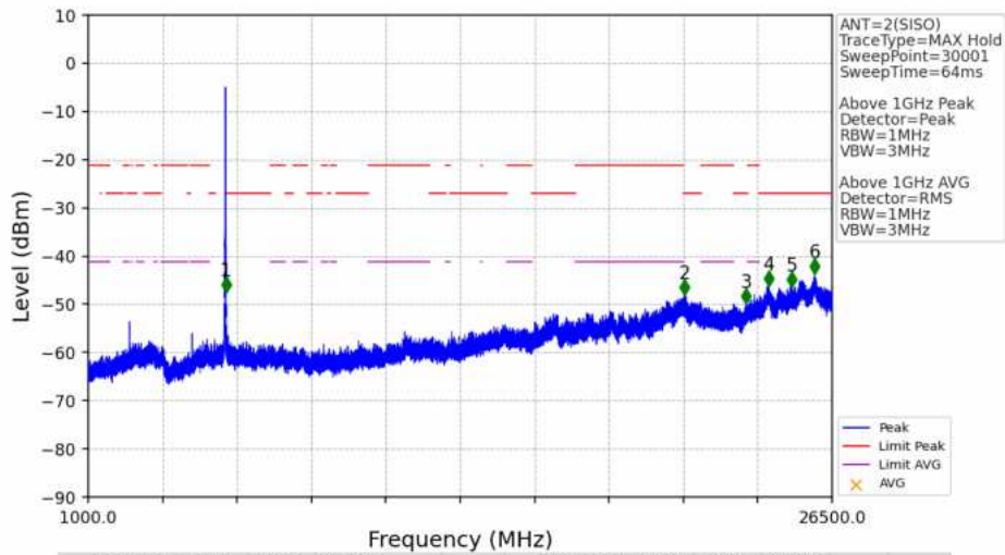
802.11a_HCH_5700MHz_Ant2_NTNV
