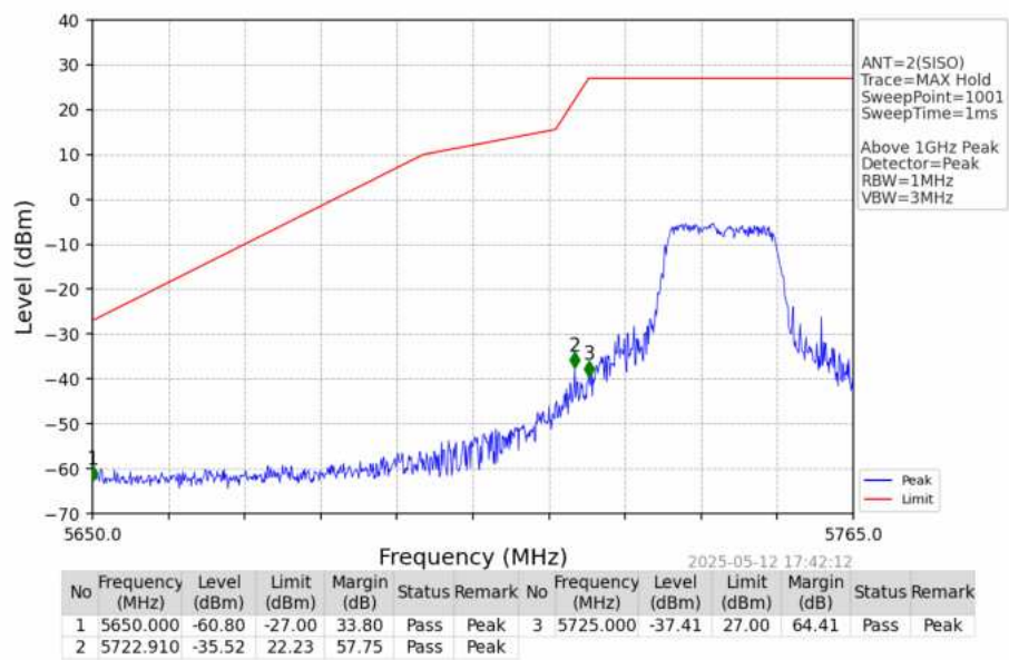
802.11a_LCH_5745MHz_Ant2_NTNV
