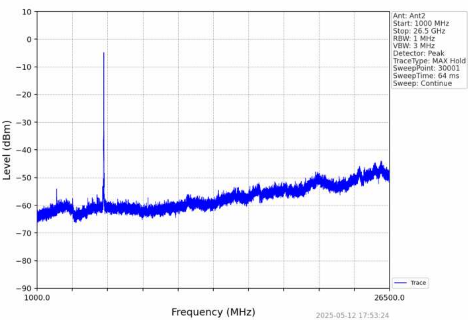
802.11a_HCH_5825MHz_Ant2_NTNV
