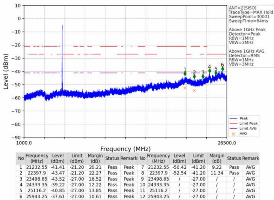
802.11a_MCH_5785MHz_Ant2_NTNV
