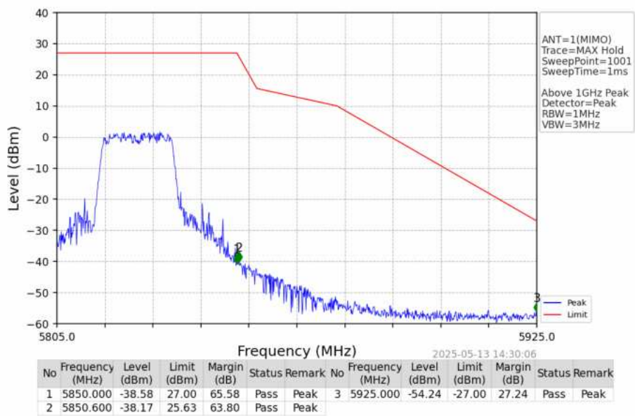
802.11n(HT20)_HCH_5825MHz_Ant1_NTNV
