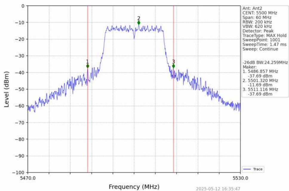
802.11a_LCH_5500MHz_Ant2_NTNV
