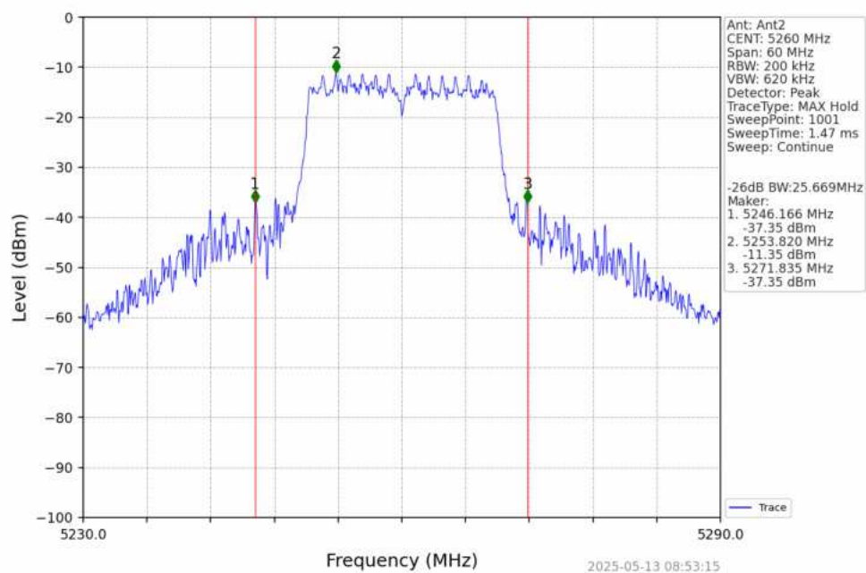
802.11n(HT20)_LCH_5260MHz_Ant2_NTNV
