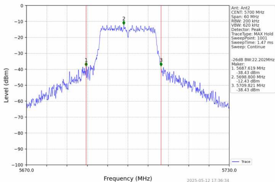
802.11a_HCH_5700MHz_Ant2_NTNV
