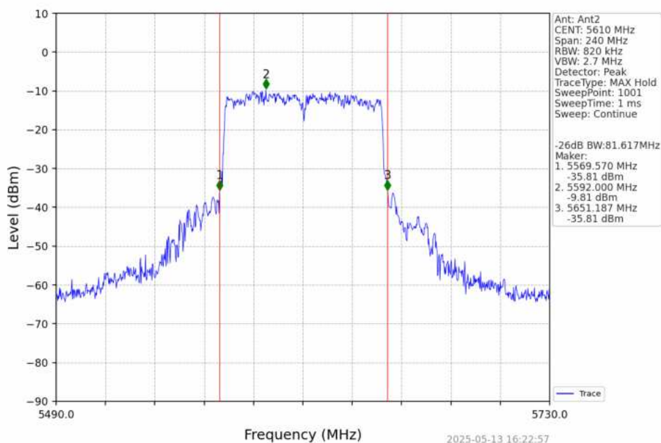
802.11ac(VHT80)_HCH_5610MHz_Ant2_NTNV
