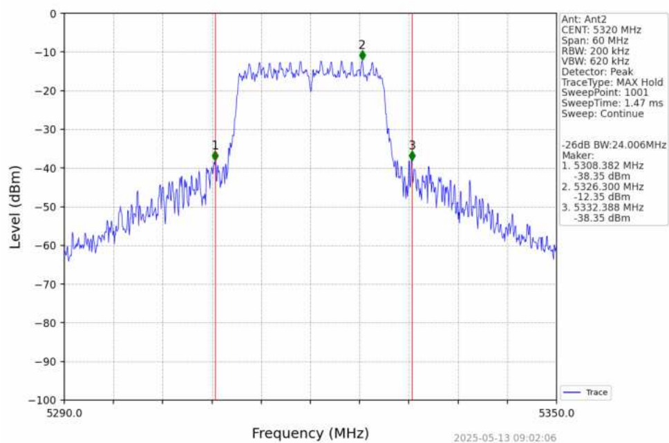
802.11n(HT20)_HCH_5320MHz_Ant2_NTNV
