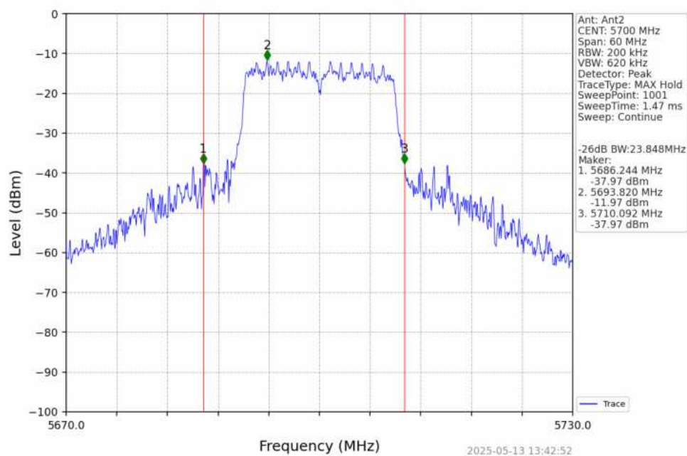
802.11n(HT20)_HCH_5700MHz_Ant2_NTNV
