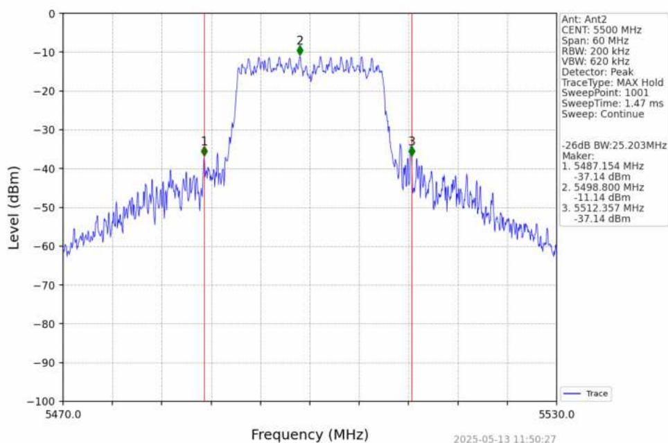
802.11n(HT20)_LCH_5500MHz_Ant2_NTNV
