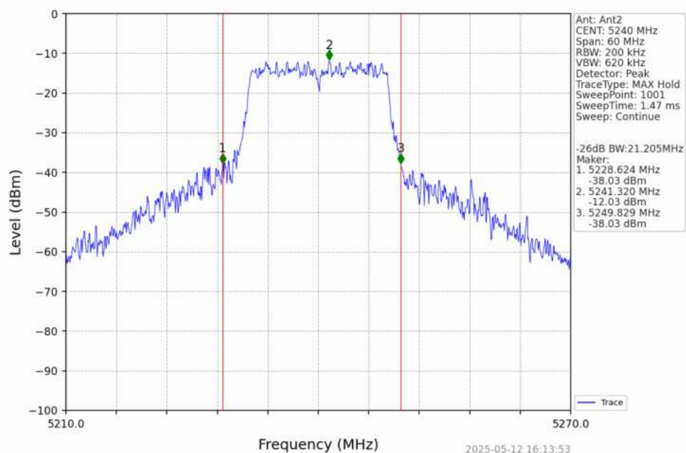
802.11a_HCH_5240MHz_Ant2_NTNV
