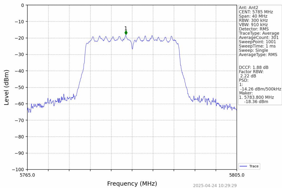
802.11n(HT20)_MCH_5785MHz_MIMO_NTNV
