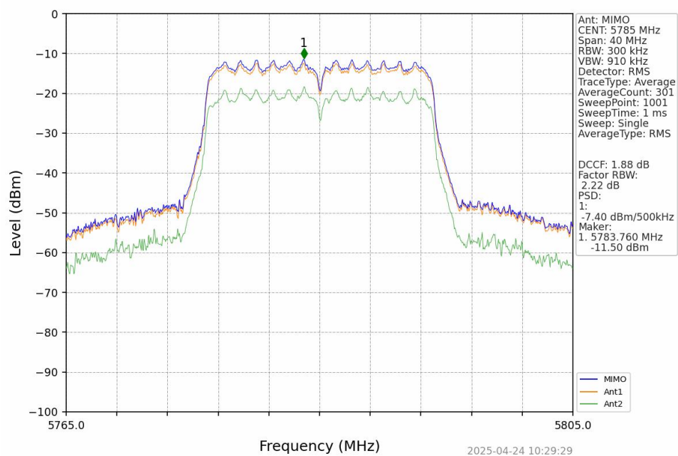
802.11n(HT20)_MCH_5785MHz_MIMO_NTNV
