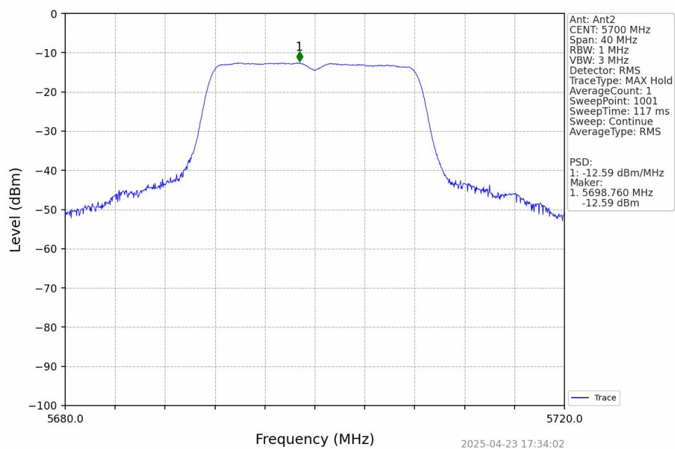
802.11a_HCH_5700MHz_Ant2_NTNV
