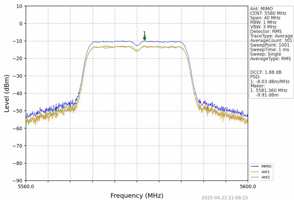
802.11n(HT20)_MCH_5580MHz_MIMO_NTNV
