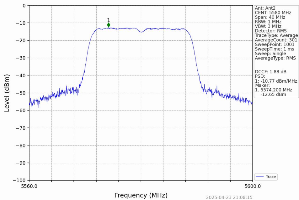
802.11n(HT20)_MCH_5580MHz_MIMO_NTNV
