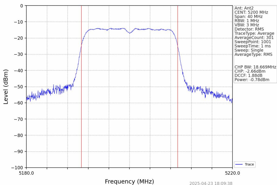
802.11n(HT20)_MCH_5200MHz_Ant2_NTNV
