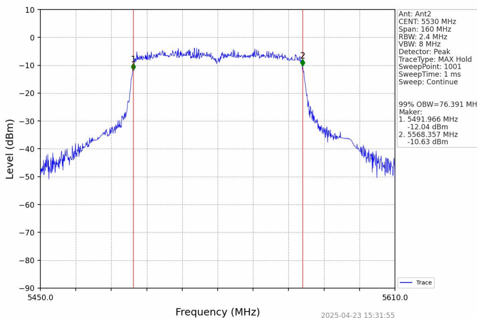
802.11ac(VHT80)_LCH_5530MHz_Ant2_NTNV
