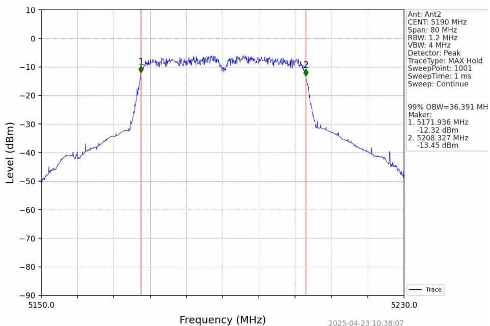
802.11n(HT40)_LCH_5190MHz_Ant2_NTNV
