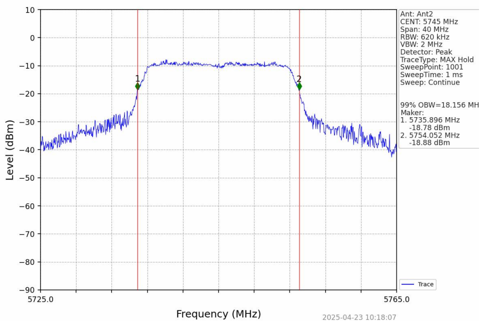
802.11a_LCH_5745MHz_Ant2_NTNV
