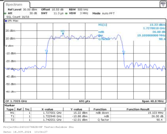
26%OBW Band 4 20MHz/1732.5/Mid QPSK 100@0
