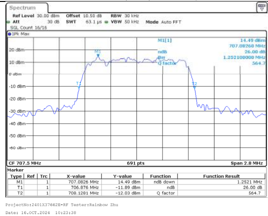
26%OBW Band 12 1.4MHz/707.5/Mid 16QAM 6@0
