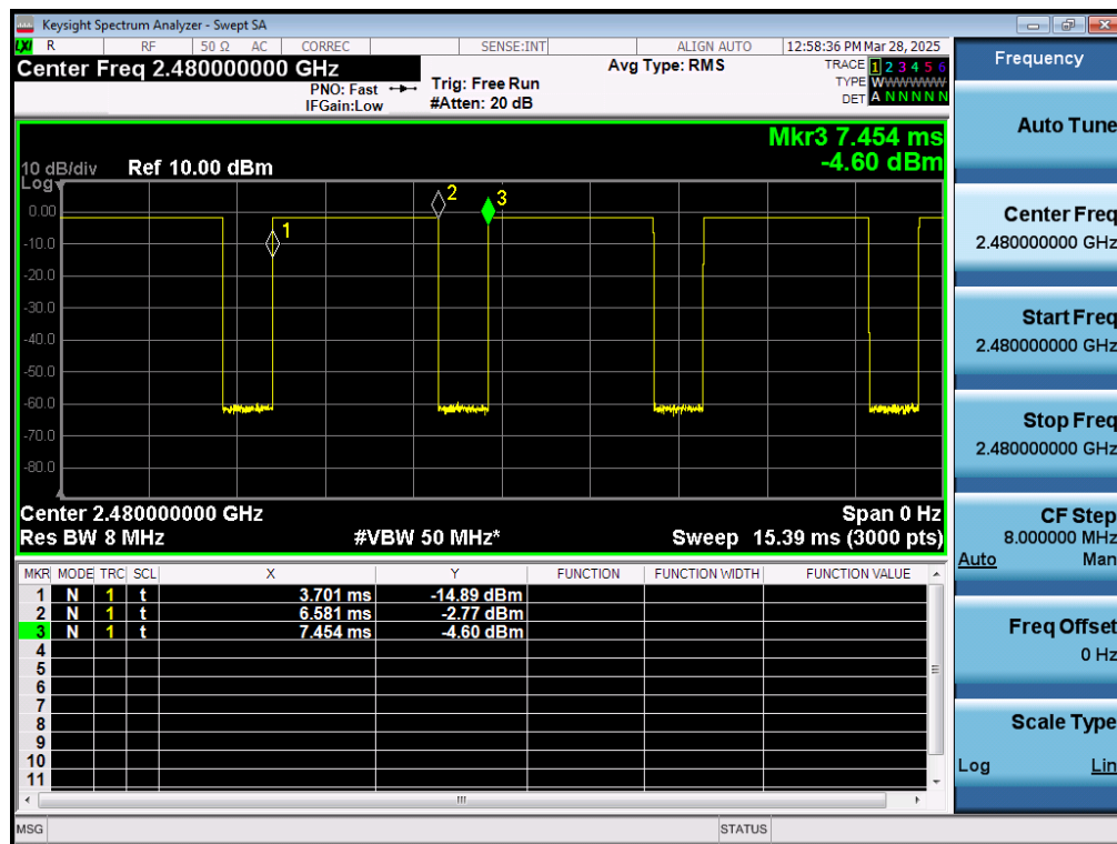
BR-GFSK-ANT1-2480
