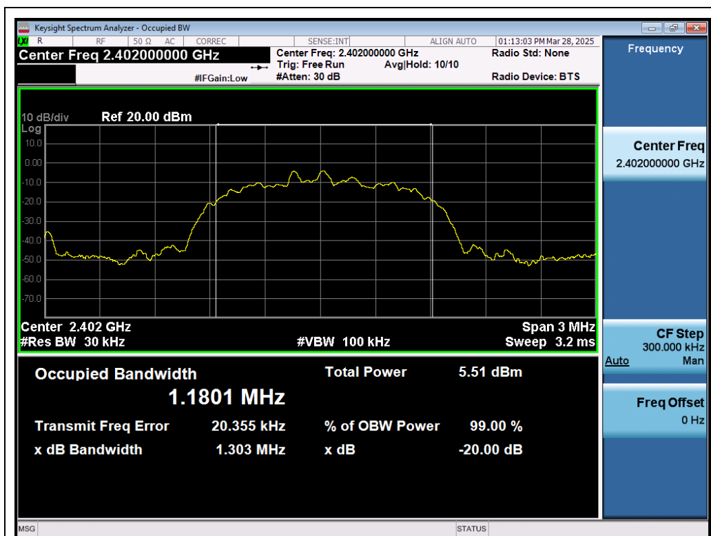
Test_Graph_EDR_ANT1_2402_3Mbps_OBW
