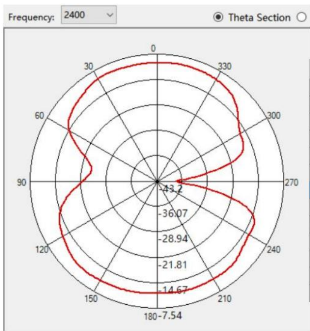
Vertical:2400MHz
