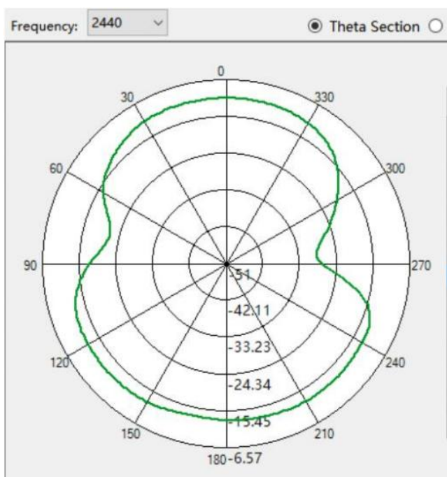
Vertical:2440MHz
