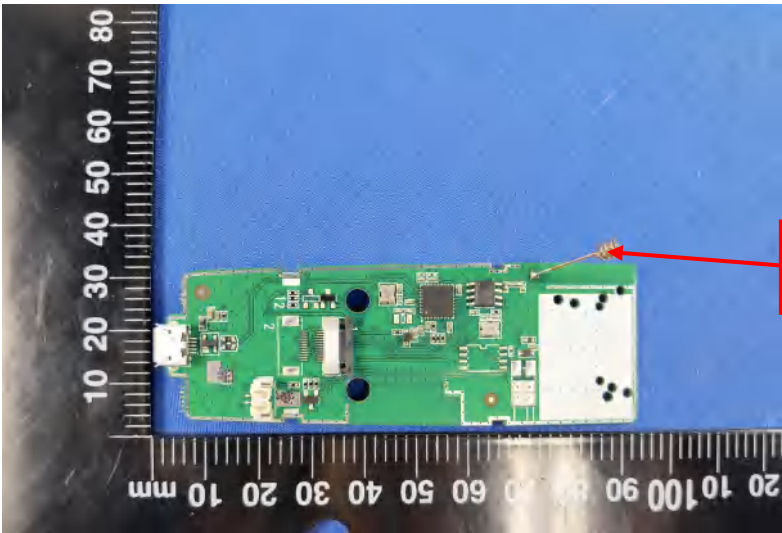
2.4G Antenna
