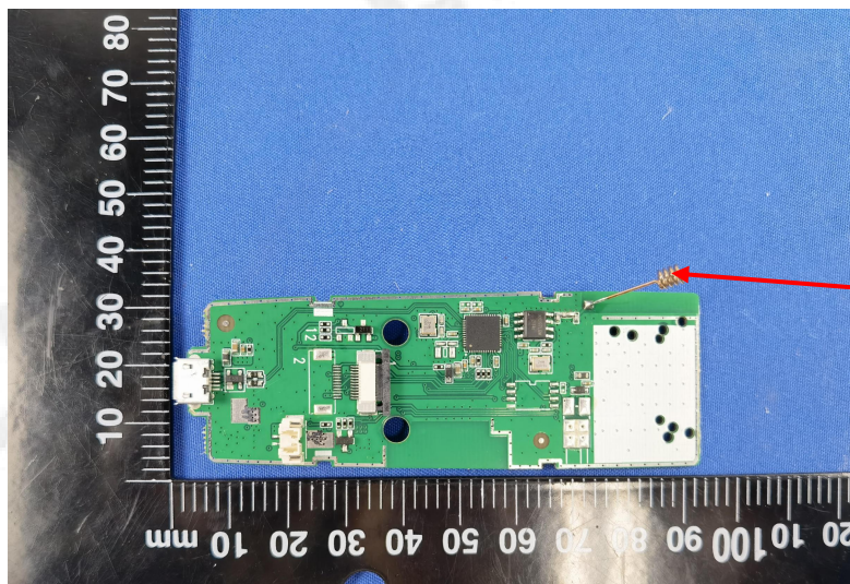
2.4G Antenna
