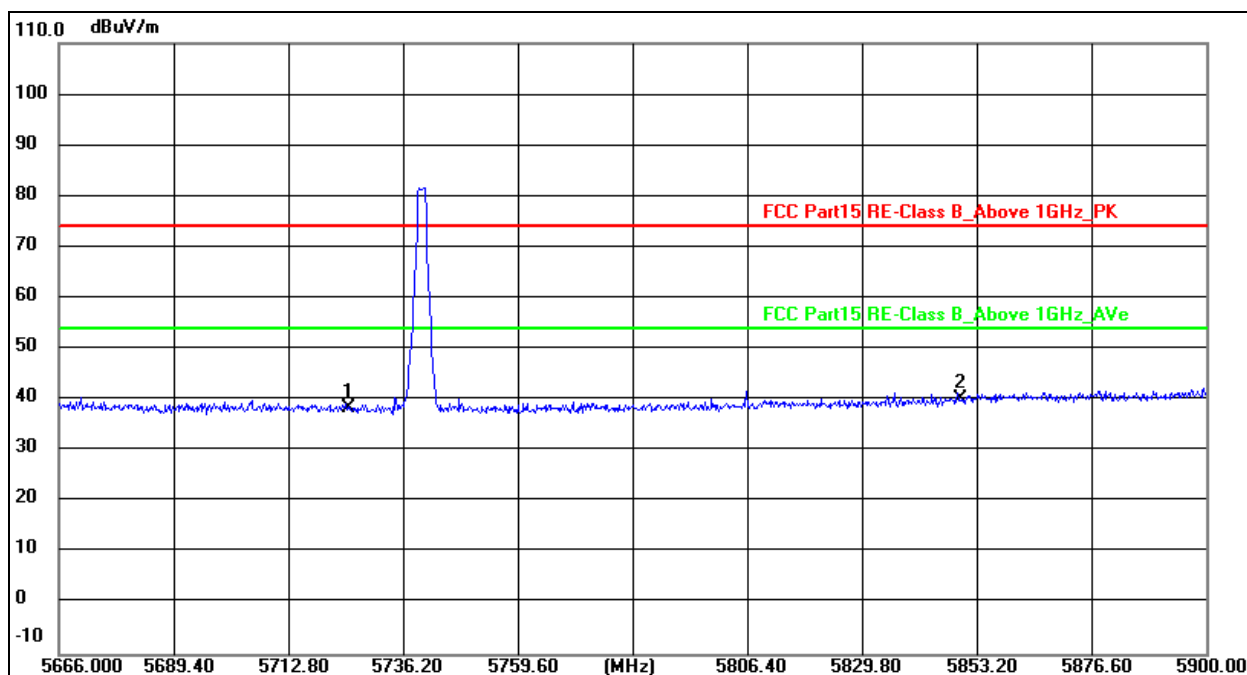
5740MHz Horizontal
