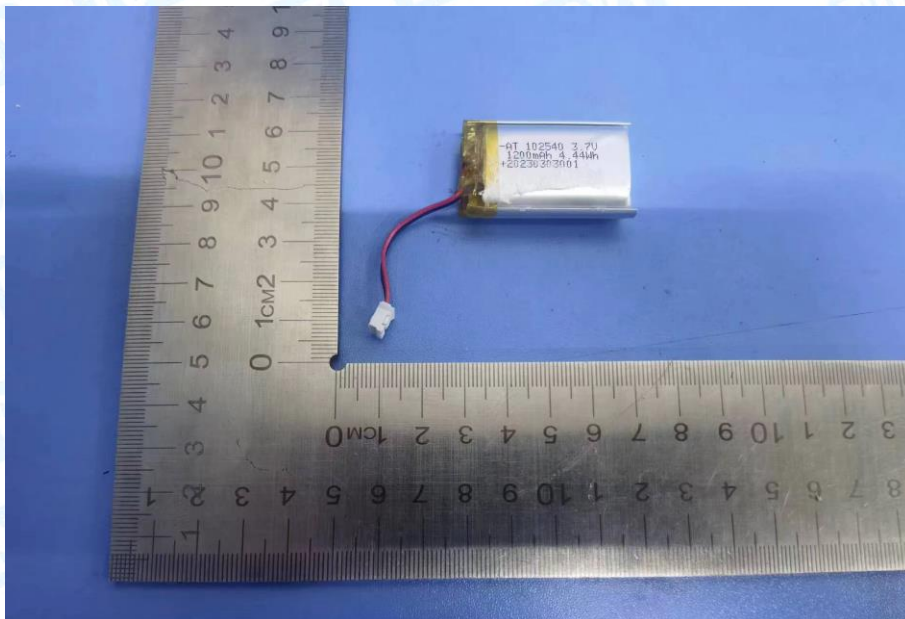
Photo 14 Battery parameters
