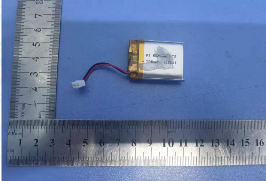
Photo 12 Battery parameters
