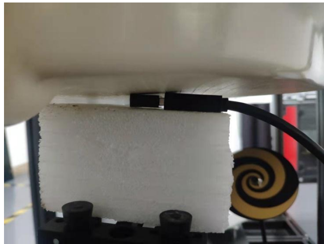
Horizontal-Up(0mm)
