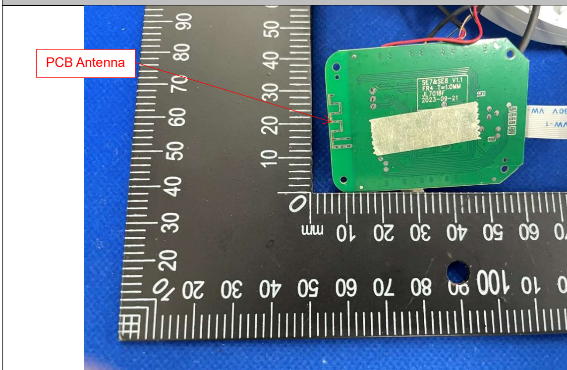
EUT Photo
